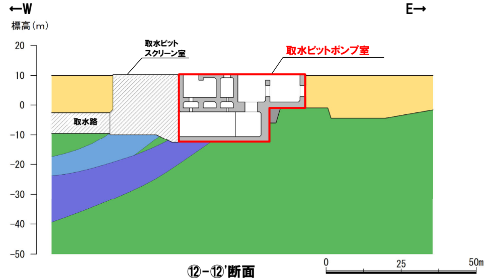
①-①'断面
