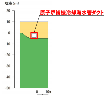
⑦-⑦'断面
