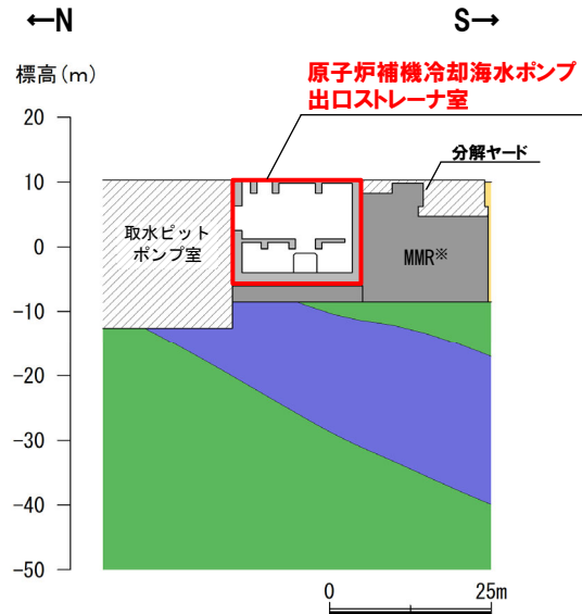
⑨-⑨'断面
