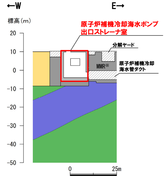
⑩-⑩'断面
