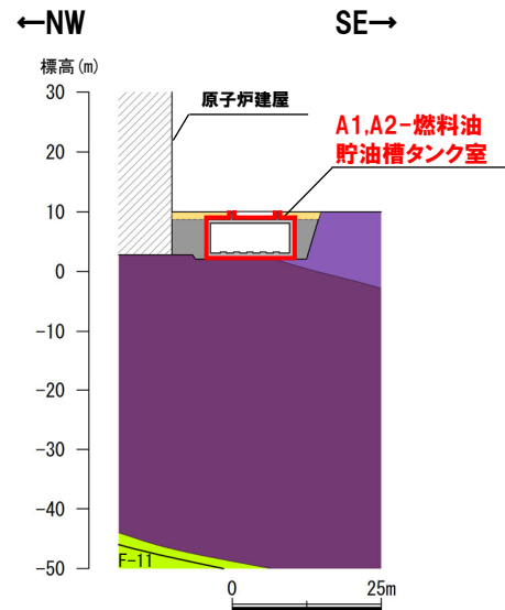
①-①'断面
