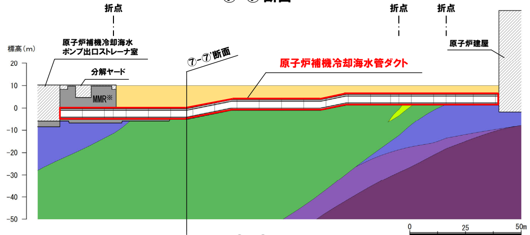
⑧-⑧'断面
