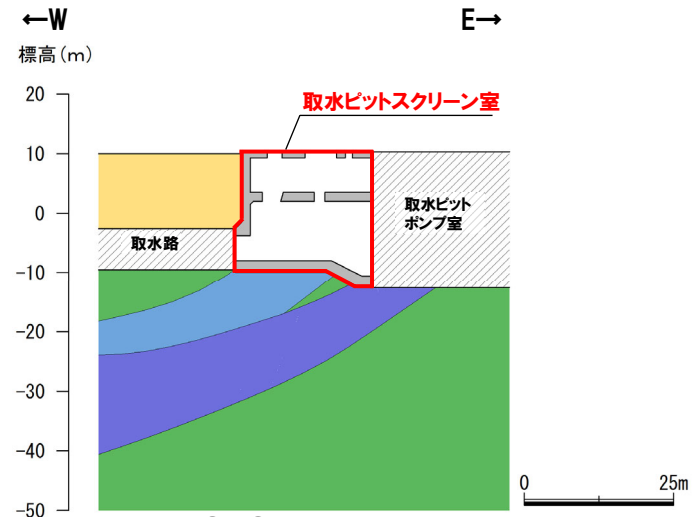
⑭-⑭'断面
