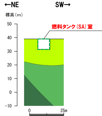
②③-②③' 断面
