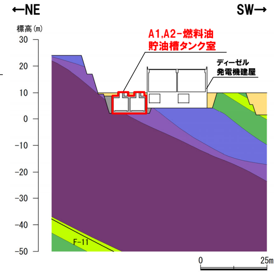
②-②'断面
