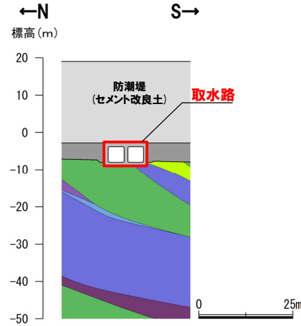
17-17' 断面
