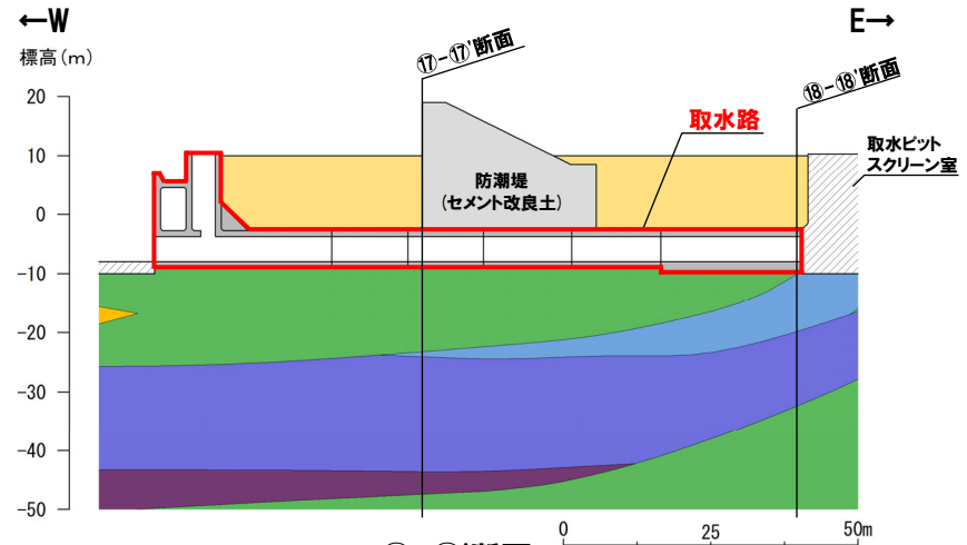
19-19' 断面
