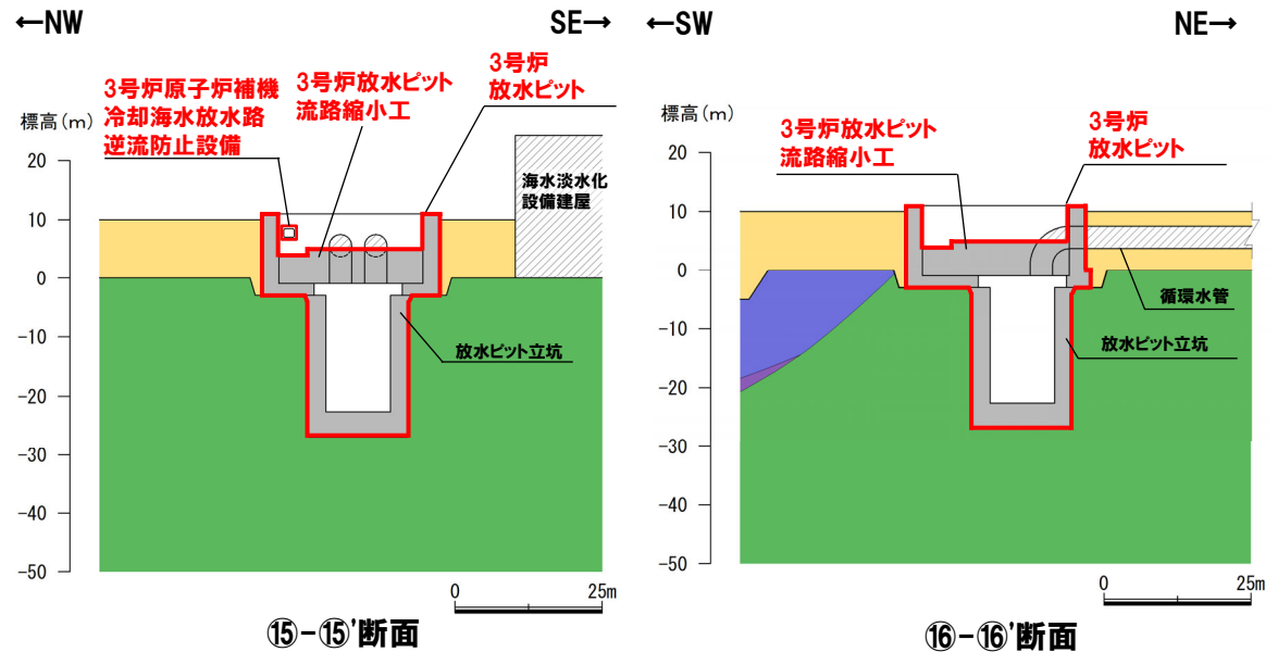
3号炉放水ピット等断面図
