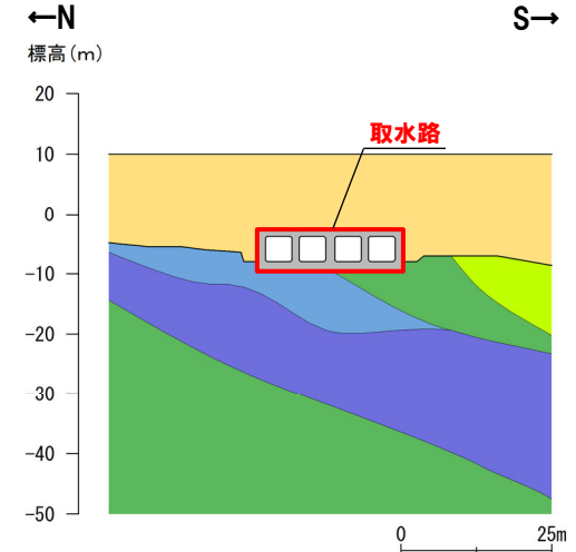
18-18' 断面
