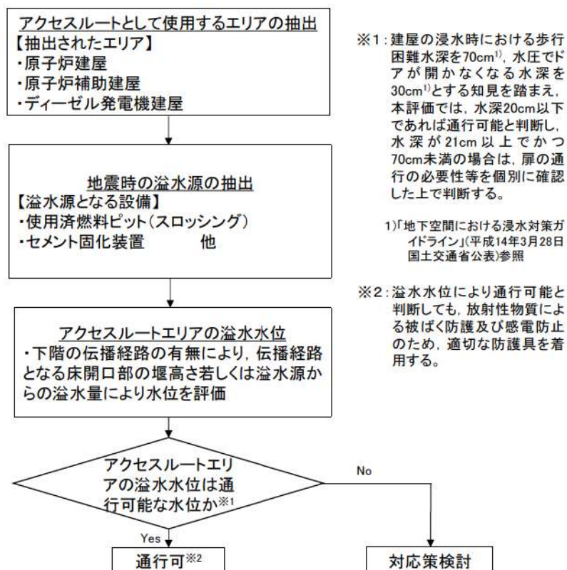
第1図 地震発生による内部溢水時のアクセサルート評価フロー
