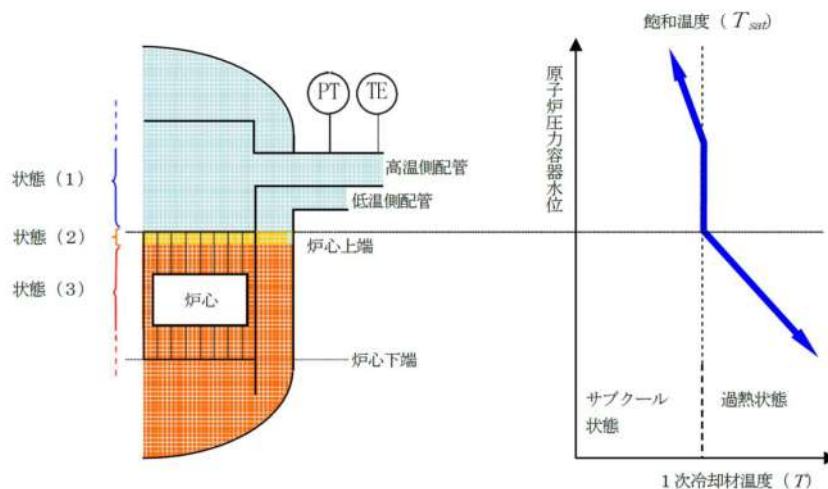
第5図 原子炉圧力容器内の水位と水位変化の概念図
