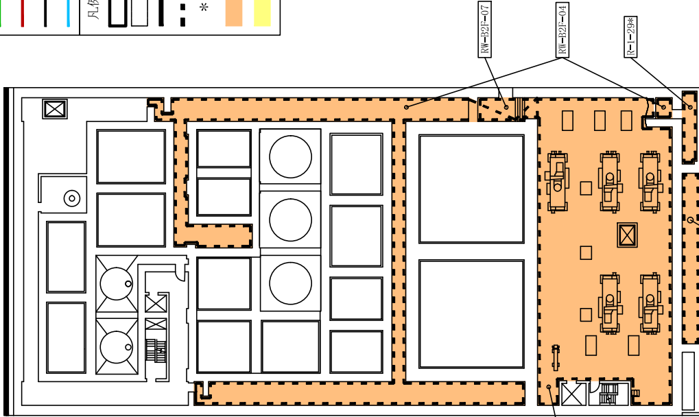
廃棄物処理建屋 T. M. S. L. -1100
