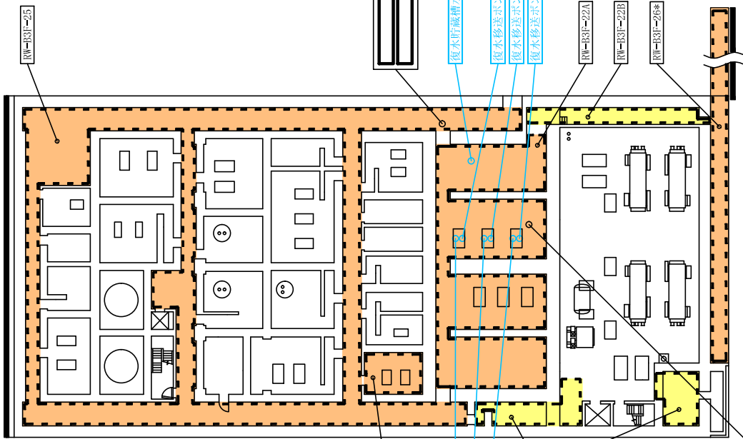
廃棄物処理建屋 T. M. S. L. -6100
