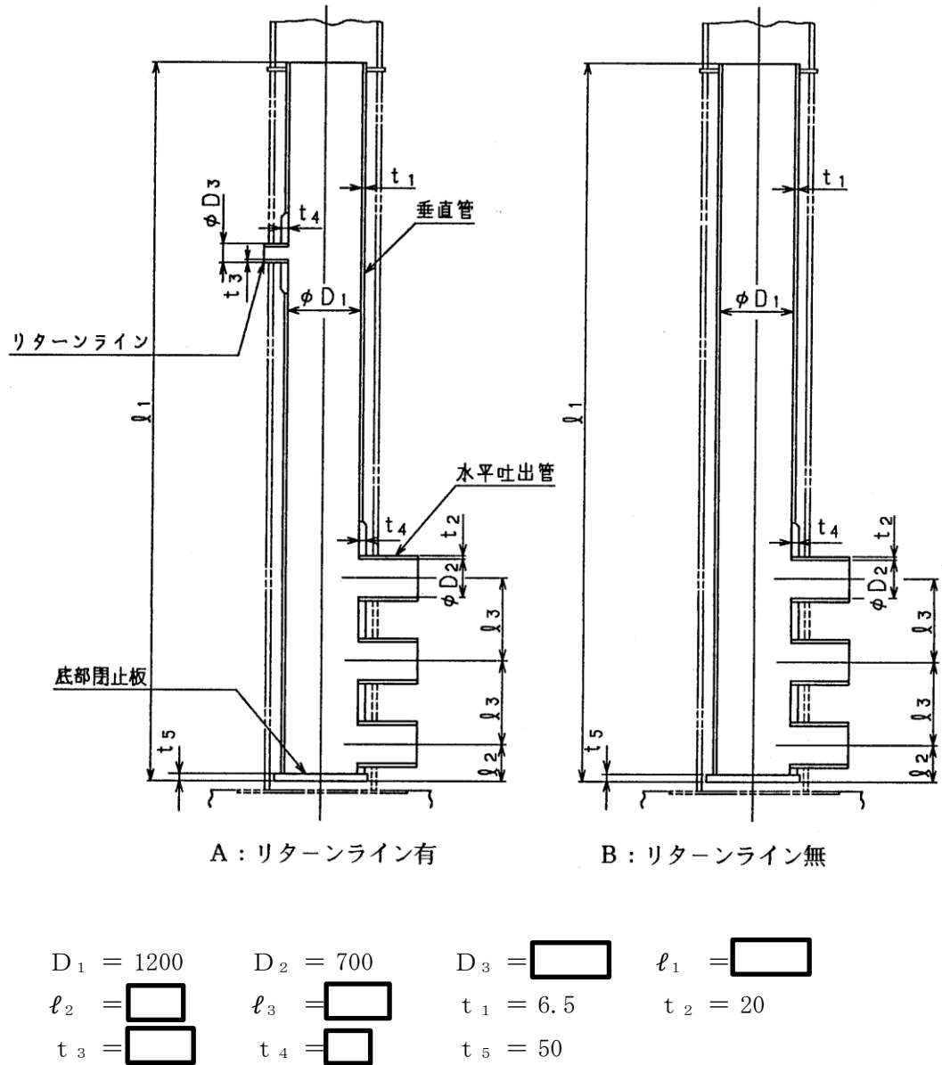
図3-1 ベント管の形状及び寸法 (単位: mm)
