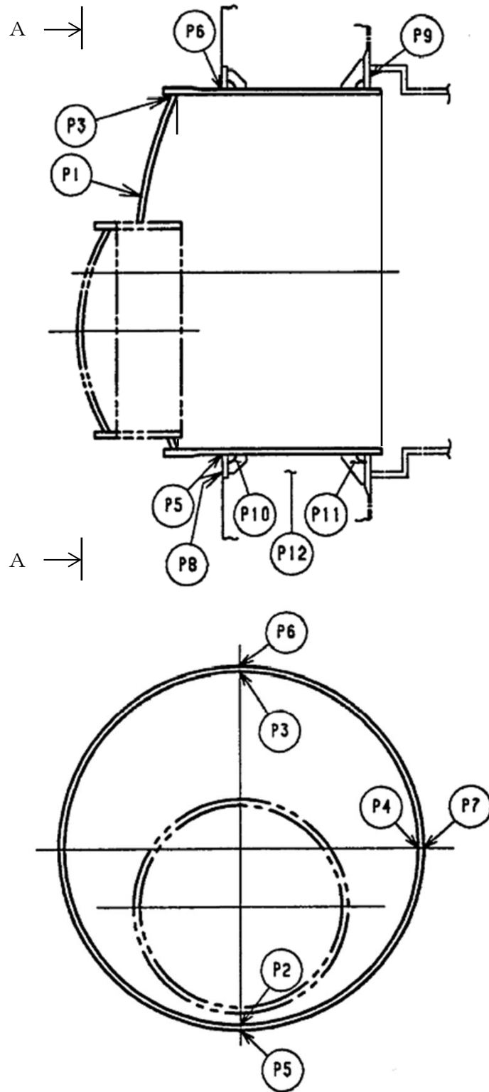
A~A矢视图
