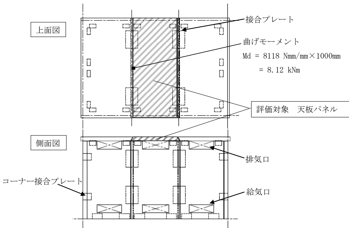
図 1.2-9 天板パネル
