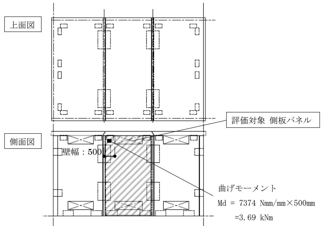
図 1.2-5 側板パネル
