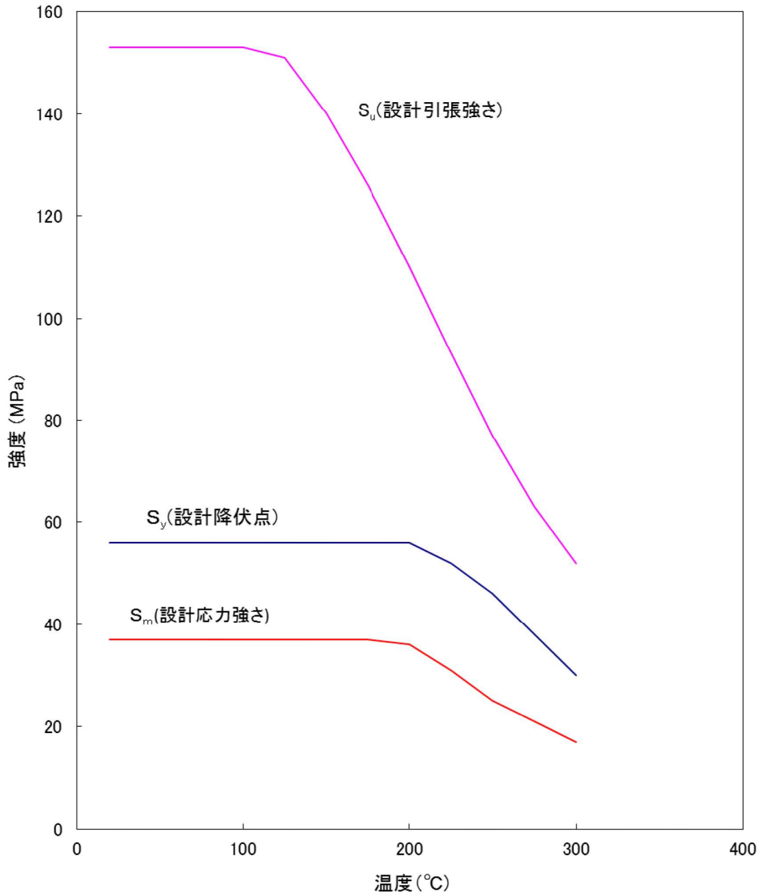
(甲)-第 A. 8 図 アルミニウム合金 (MB-A3004-H112) の 温度に対する機械的性質の変化(1/2) (注1)
