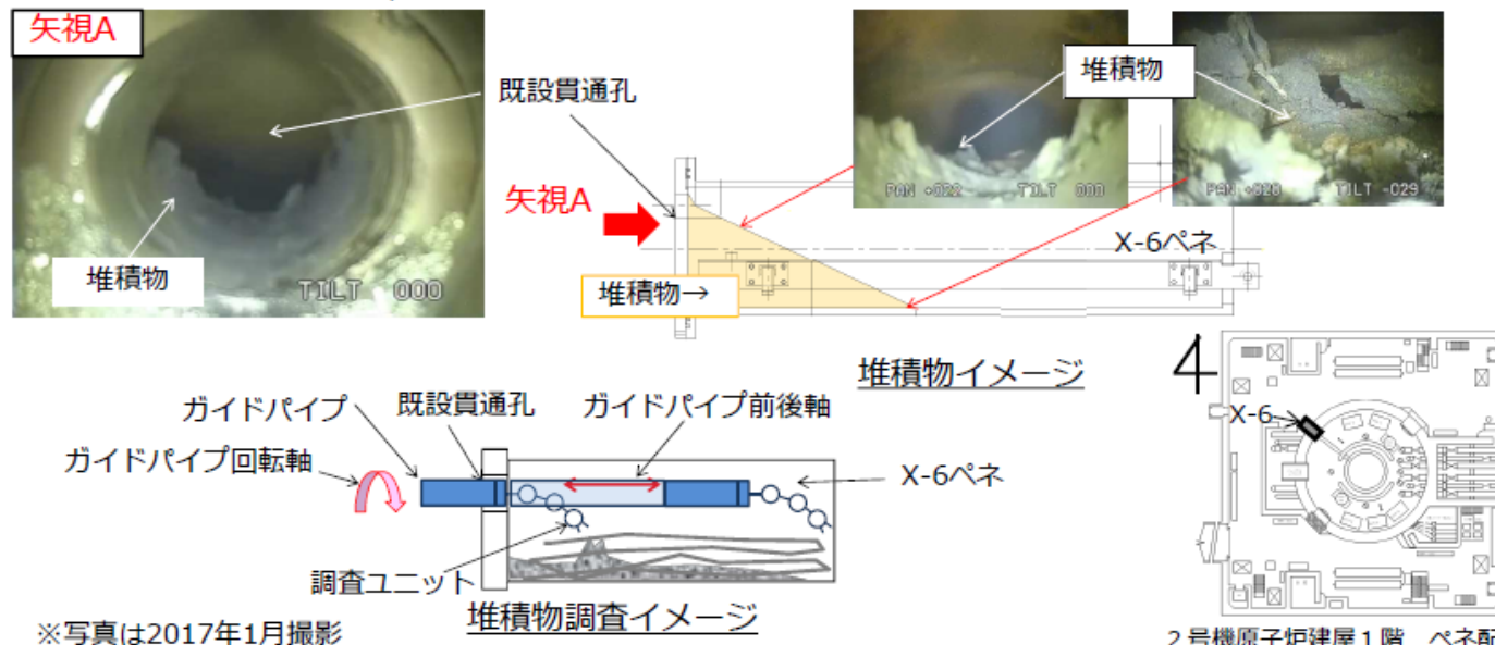
2号機原子炉建屋1階 ペネ配置図
