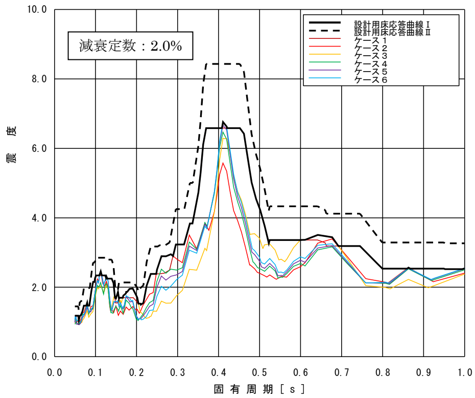
図 4-1 設計用床応答曲線の例
