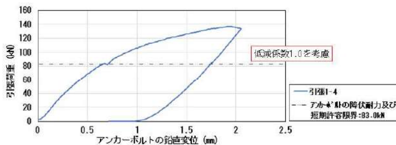
第 7-78 図 アンカーボルトの鉛直変位 (mm) (引張1-4)
