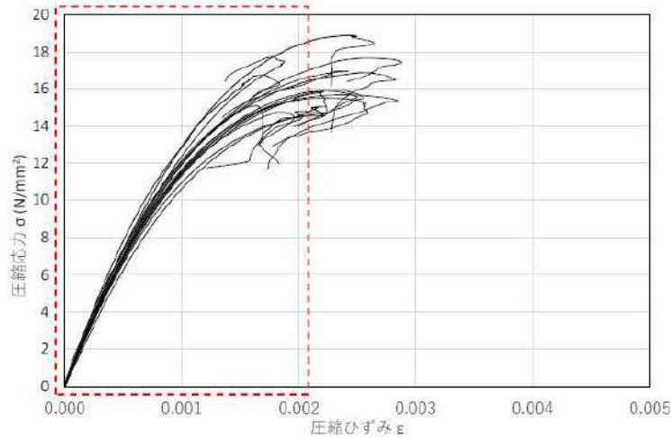
第 7-55 図 セメント改良土の一軸圧縮強度試験結果
