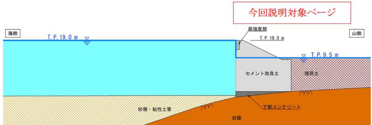
第 9-19 図 地下水位及び海側の水位の概要図（津波時）
