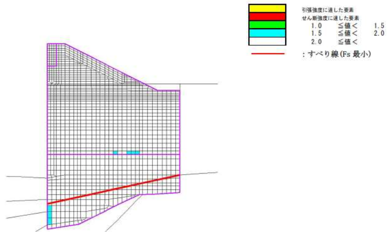
第 9-34 図 最小すべり安全率時刻時の局所安全係数分布 (地震時)
