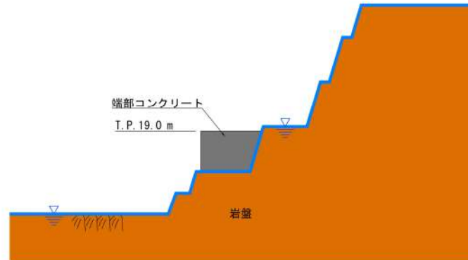
第 9-52 図 地下水位概要図（地震時）
