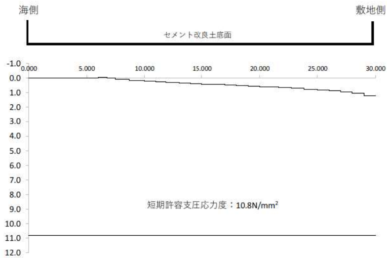
第 9-37 図 下部コンクリートの接地圧分布（津波時）
