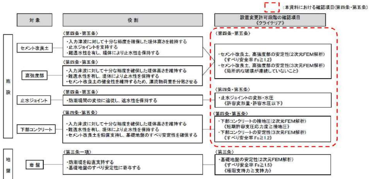
第 8-1 図 設置変更許可段階における確認項目 [防潮堤（標準部）]
