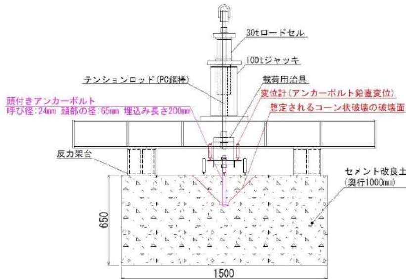
第 7-58 図 引張試験概要図 (側面図)
