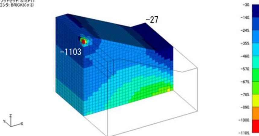
第 9-32 図 基本ケースの圧縮主応力分布図
