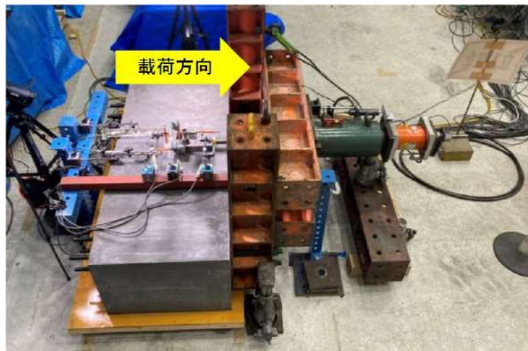
第 7-61 図 せん断試験イメージ写真
