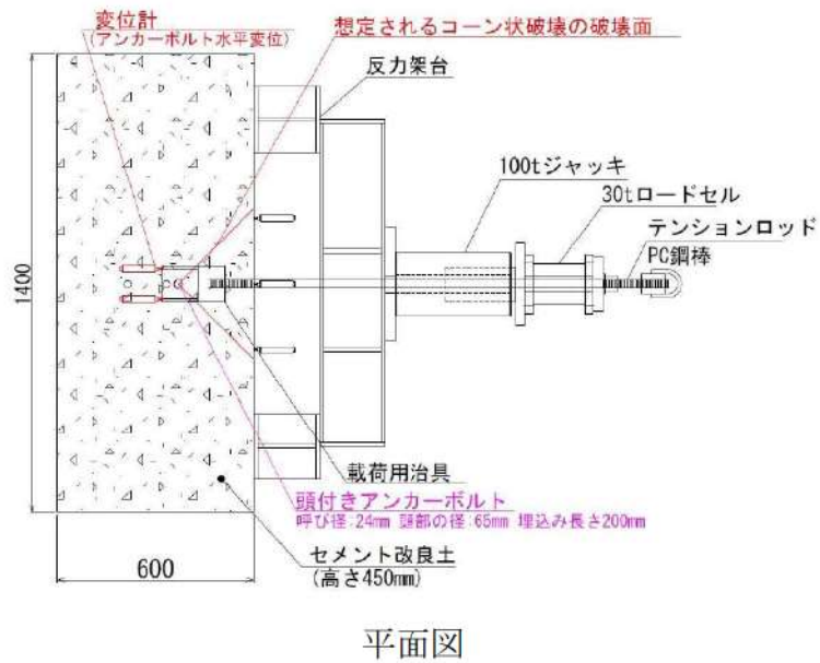
第 7-60 図 せん断試験概要図
