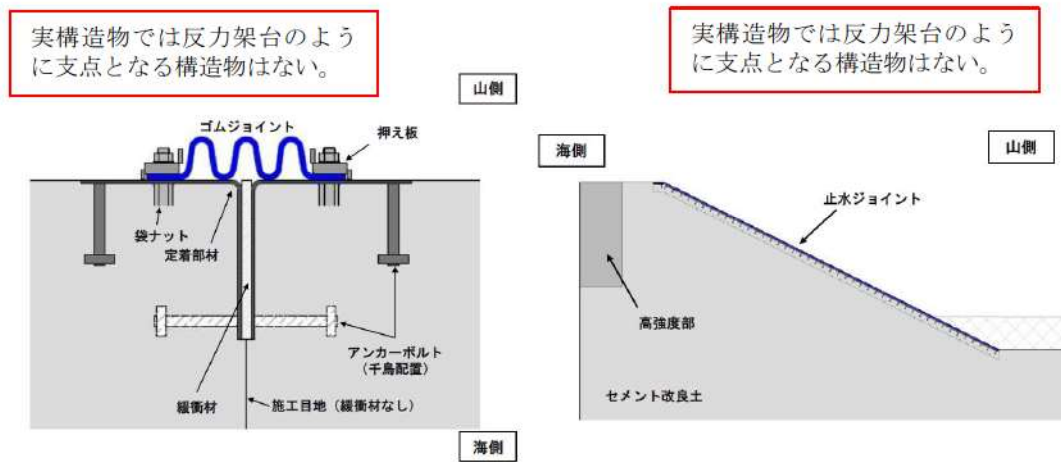
第 7-77 図 防潮堤イメージ図
