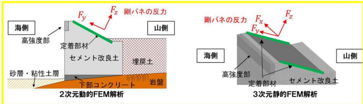
第 9-41 図 剛バネの反力 ( F_x , F_y , F_z )
