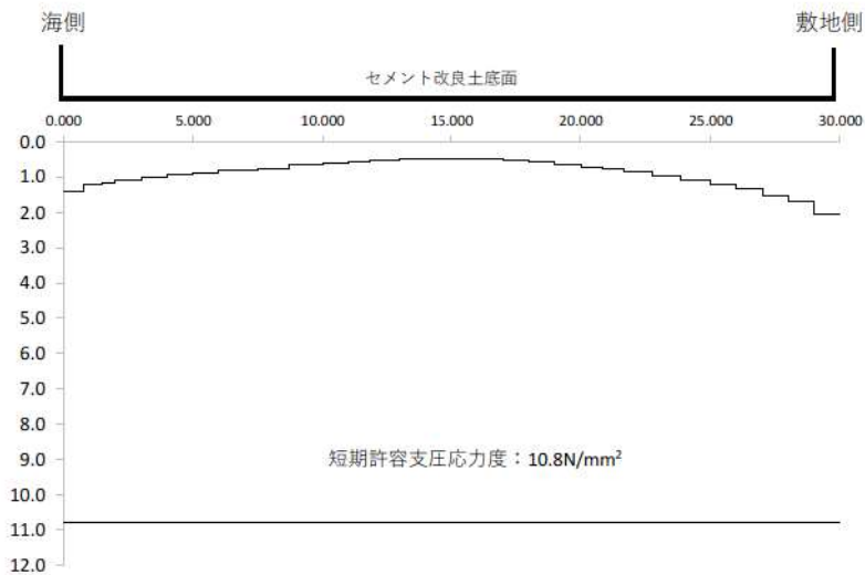
第 9-39 図 下部コンクリートの接地圧分布（重畳時）
