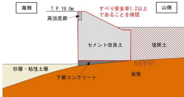
第9-21図 2次元動的FEM解析での確認概要
