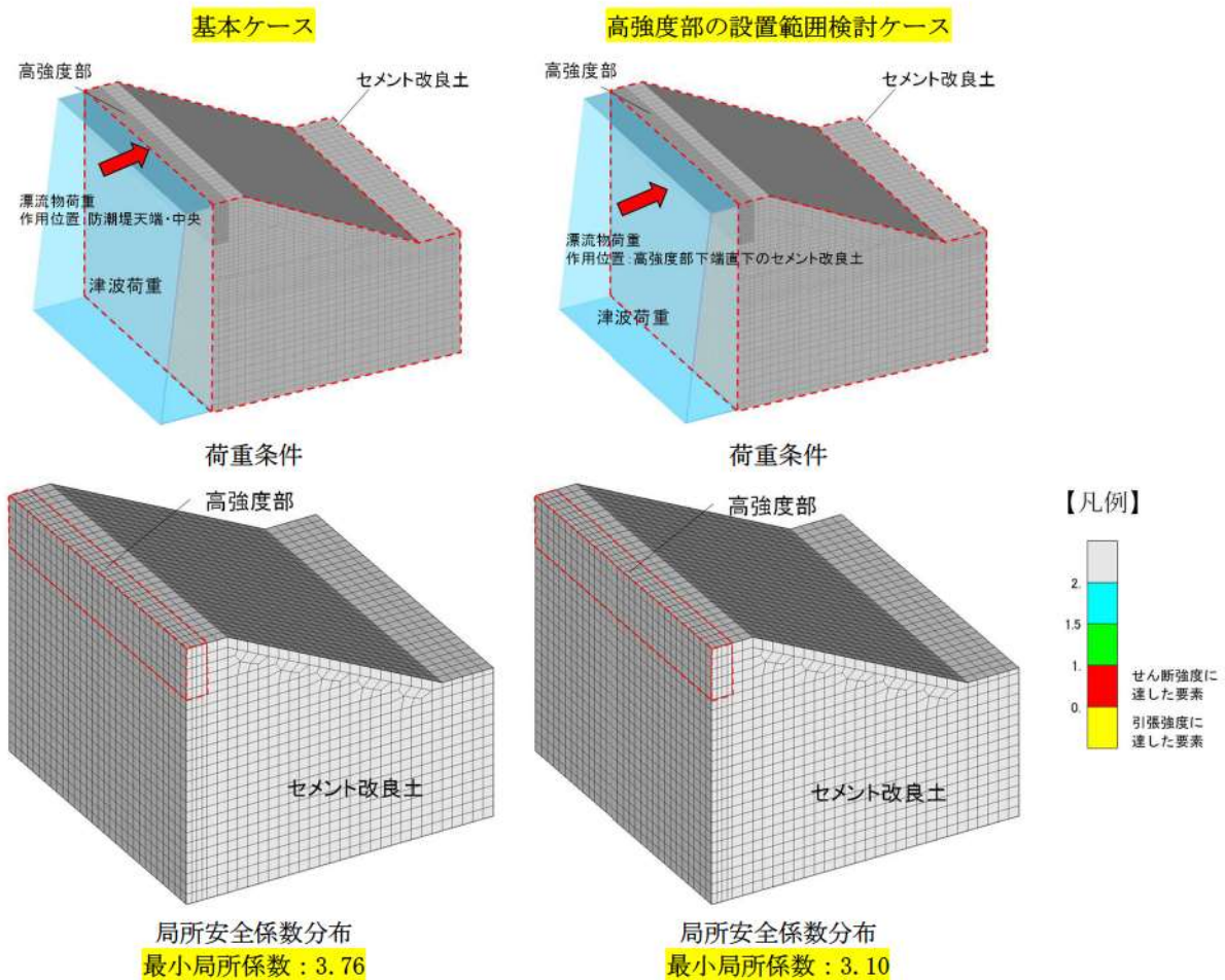
第 9-31 図 局所安全係数分布 (津波時)
