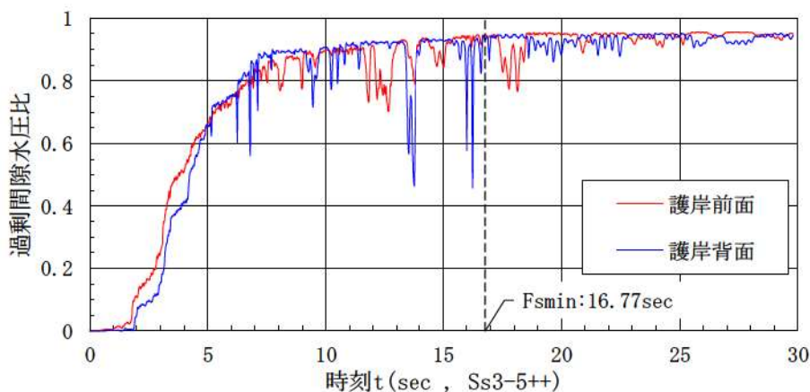
第 9-30 図 防潮堤背面の着目要素における過剰間隙水圧比の時刻歴
