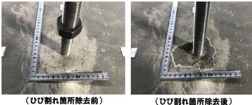
第 7-66 図 引張試験1-4 引張試験後の状況写真
