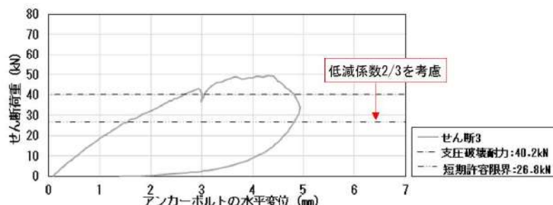
第 7-79 図 アンカーボルトの水平変位 (mm) (せん断3)
