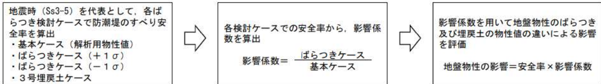
第 9-43 図 地盤物性のばらつき影響検討フロー
