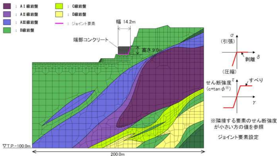
第 9-50 図 解析モデル及びジョイント要素の設定
