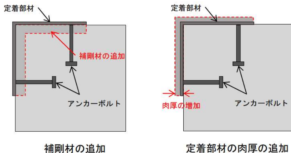
第 7-80 図 定着部材の裕度向上対策のイメージ図
