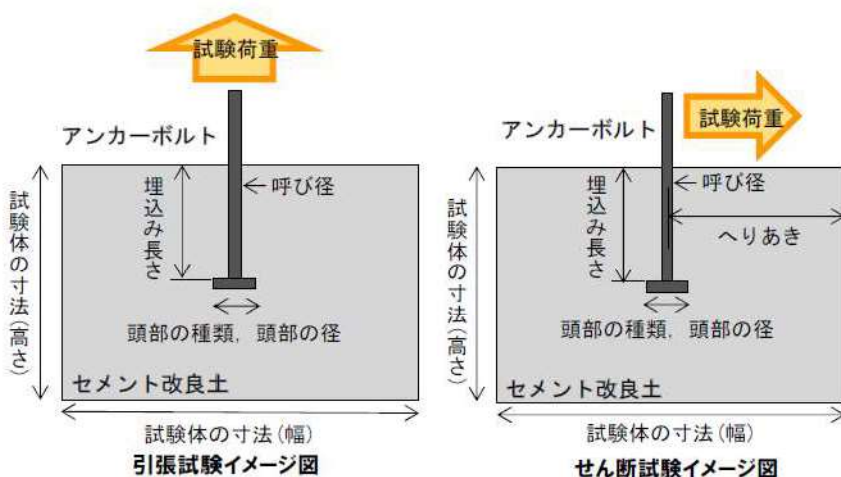
第 7-57 図 アンカーボルトの性能試験のイメージ図
