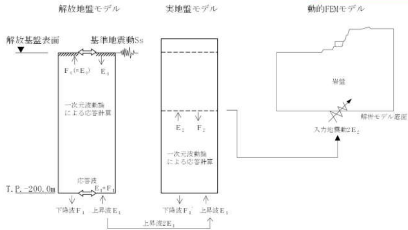
第 9-51 図 解析モデル及びジョイント要素の設定
