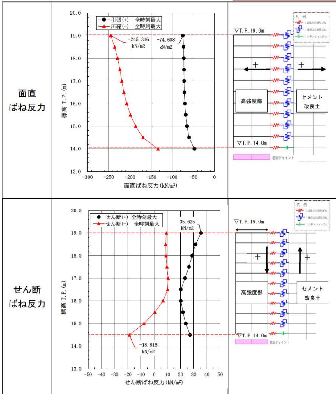
第 9-40 図 高強度部とセメント改良土の境界面（鉛直方向）に生じる引張力とせん断力の分布図
