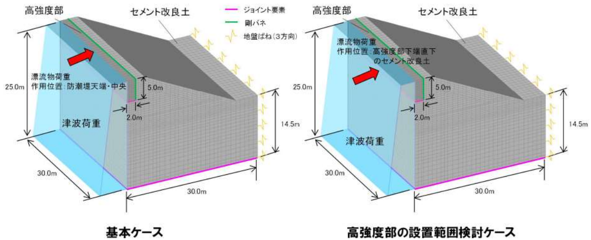
第 9-18 図 解析モデル及びジョイント要素の設定
