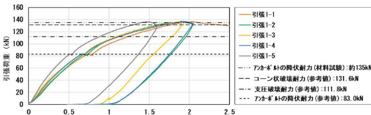
第 7-63 図 アンカーボルトの鉛直変位 (mm)
