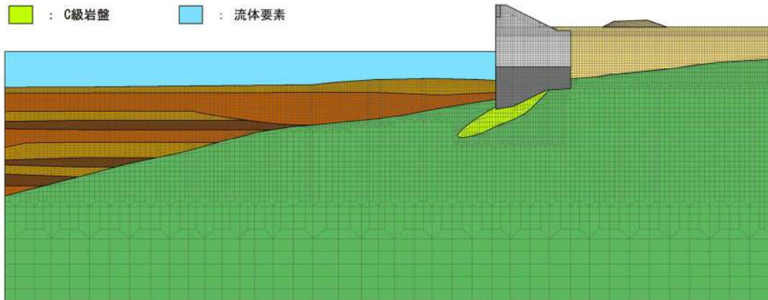
第 9-44 図 検討ケース
