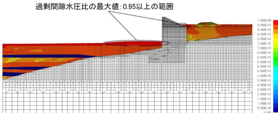
第 9-29 図 全時刻最大の過剰間隙水圧比の分布図
