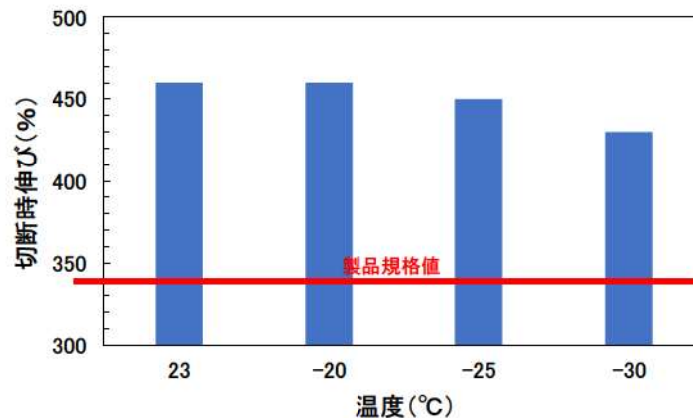
第 3-5 図 ゴム材料の低温引張試験結果
