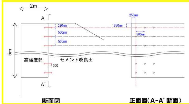
第 9-14 図 高強度部の範囲及びアンカーボルトの配置計画図
