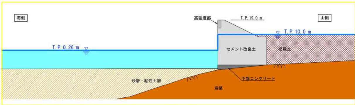
防潮堤（標準部）
