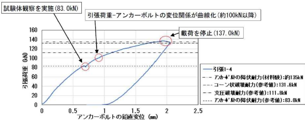
第 7-64 図 アンカーボルトの鉛直変位 引張1-4 (mm)
