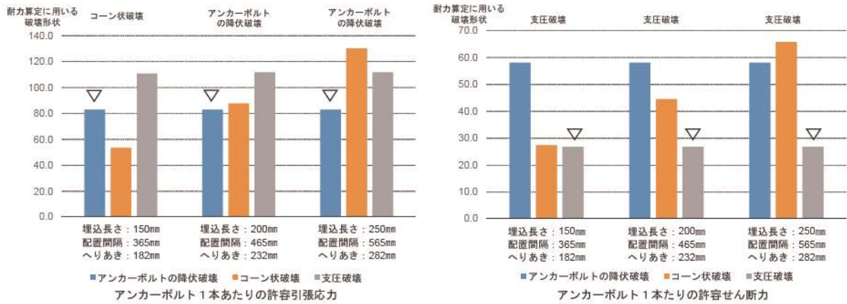
第 7-83 図 アンカーボルトの 1 本あたりの許容引張力、許容せん断耐力の計算例
