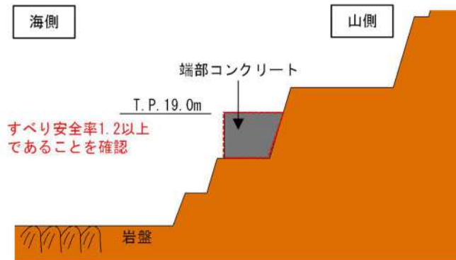
第 9-53 図 2次元動的FEM解析での確認概要
