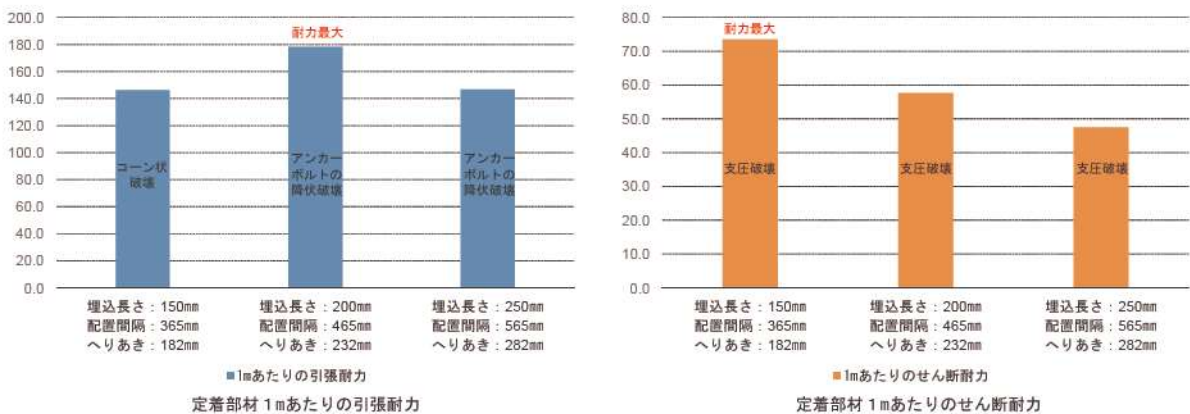
第 7-84 図 定着部材 1 mあたりの引張耐力及びせん断耐力の計算例
