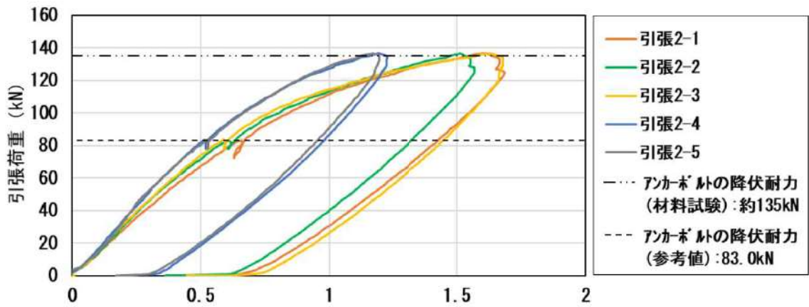
第 7-67 図 アンカーボルトの鉛直変位 (mm) (室内配合試験で確認した強度 (16.2N/mm 2 ) のケース)
