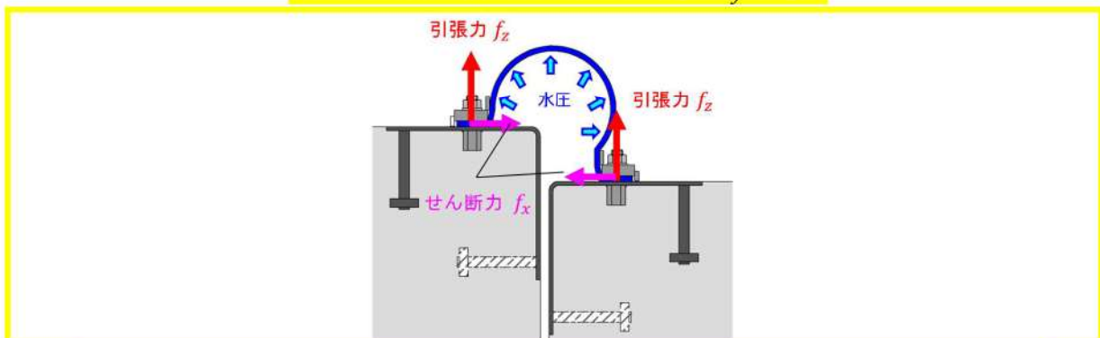
第 9-42 図 ゴムジョイントの張力により生じるせん断力 f_x ，及び引張力 f_z
