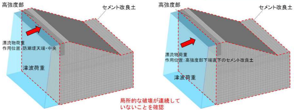
第 9-22 図 3次元静的FEM解析での確認概要
