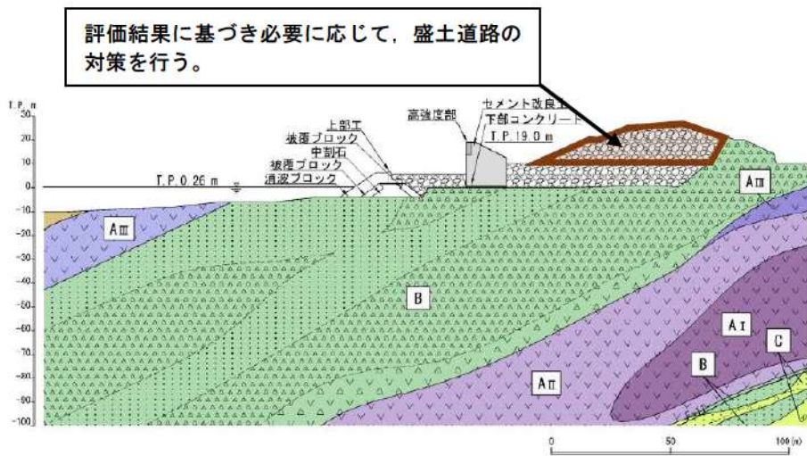
第 2-11 図 防潮堤と盛土道路の地質断面図 (5-5' 断面)
