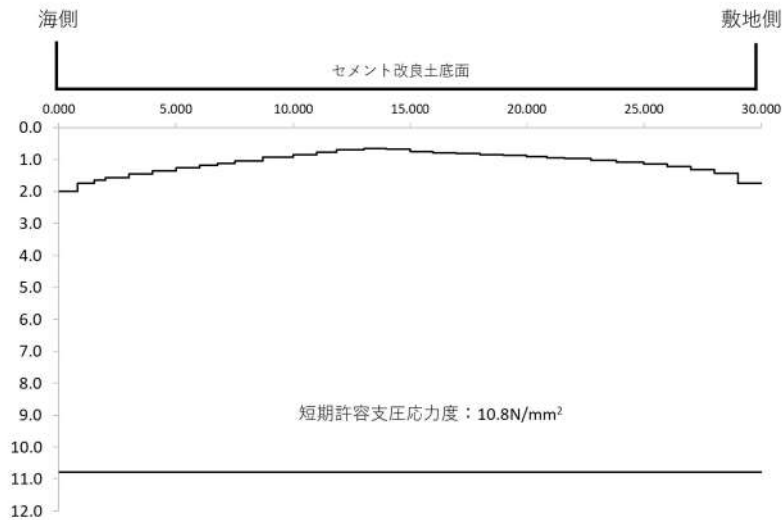
第 9-35 図 下部コンクリートの接地圧分布（地震時）
