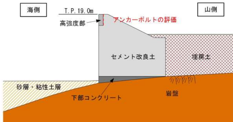
第 9-24 図 2 次元動的 F E M 解析での確認概要
