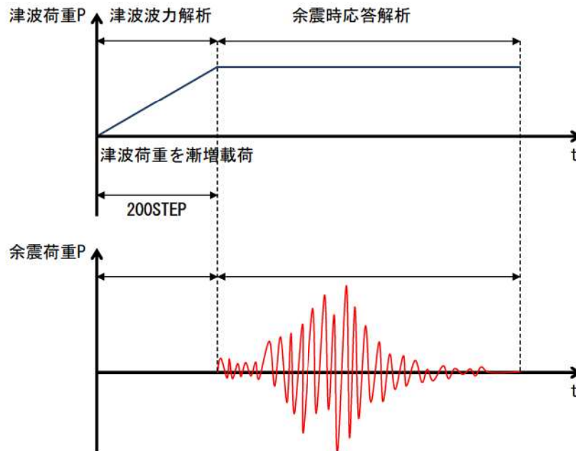
第 9-20 図 余震荷重の載荷イメージ
