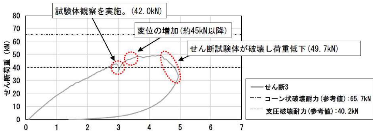
第7-69図 アンカーボルトの水平変位 せん断3 (mm)
