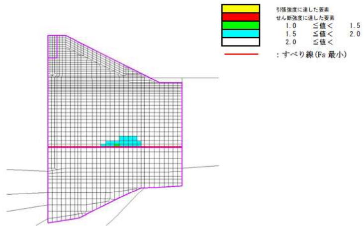
第 9-33 図 最小すべり安全率時刻時の局所安全係数分布 (重畳時)
