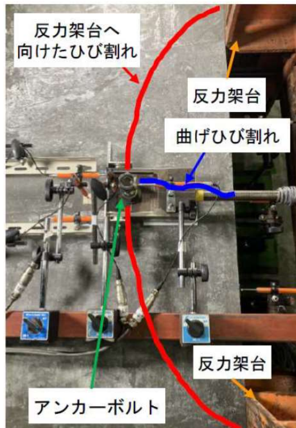
第 7-75 図 せん断試験後のひび割れ状況
