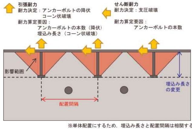
第 7-82 図 アンカーボルトの埋込み長さとは配置間隔の考え方
