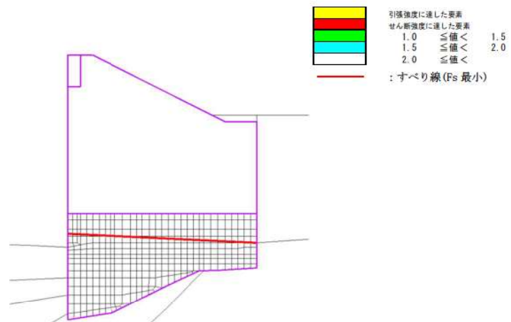
第 9-36 図 津波時の局所安全係数分布 (最小すべり線表示)
