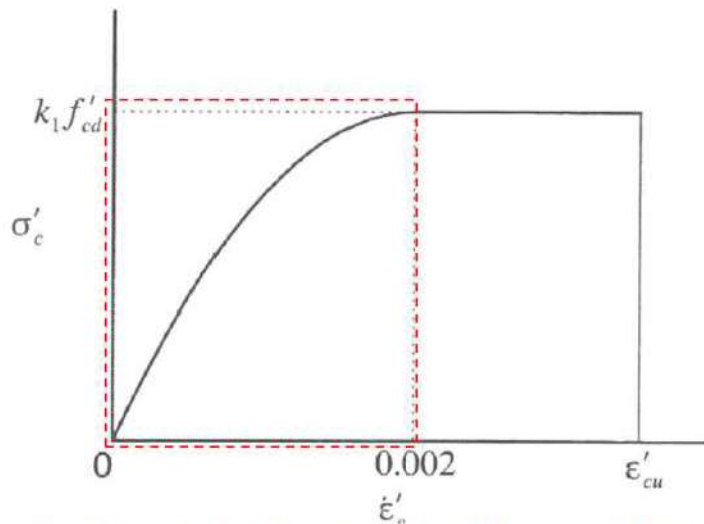
第 7-56 図 コンクリートの応力-ひずみ曲線
