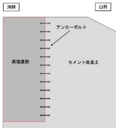
高強度部拡大図（イメージ図）
