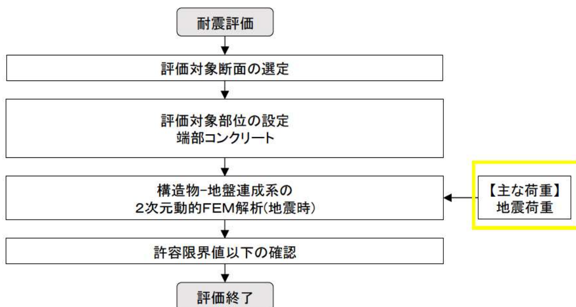
第 6-8 図 設計フロー
