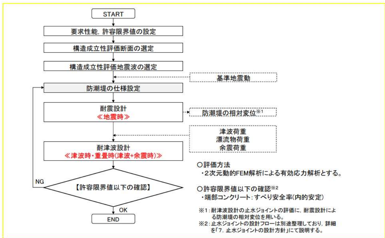
第 4-6 図 防潮堤 (端部) の設計フロー
