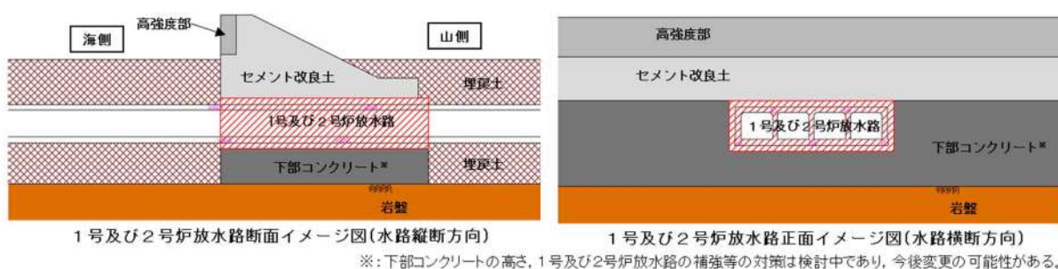
第 5-55 図 防潮堤（1号及び2号炉放水路横断部）の構造概要
