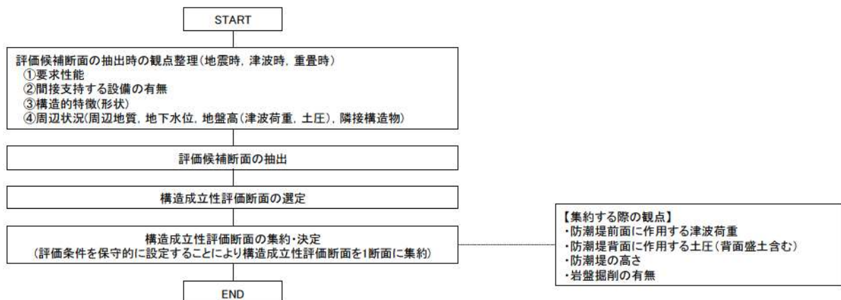
第 5-39 図 構造成立性評価断面選定フロー
