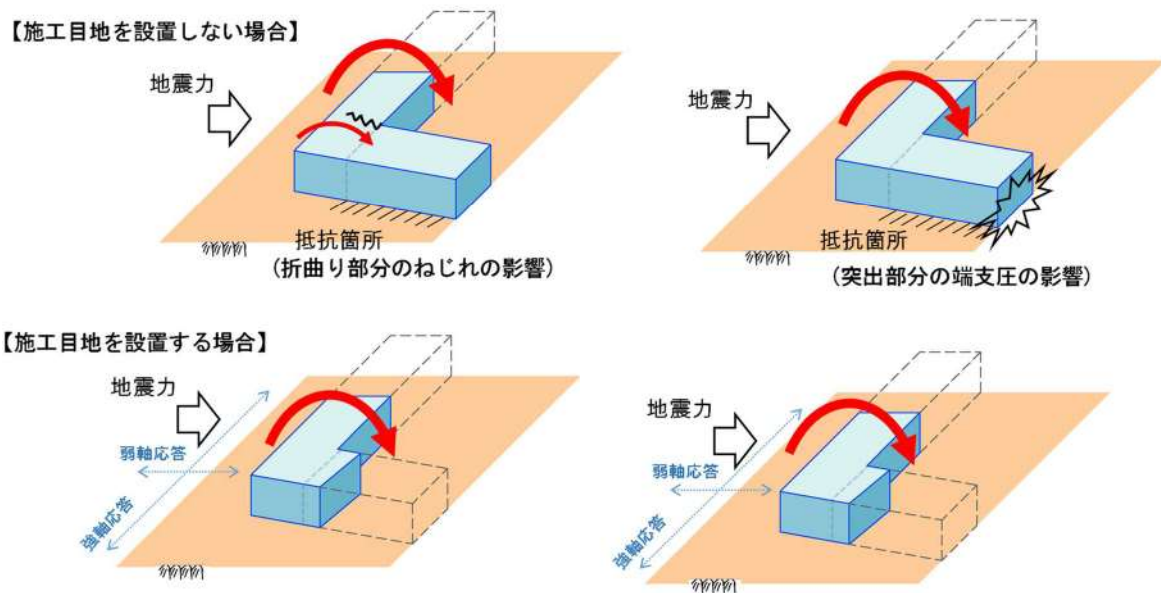
第5-44図 屈曲部形状による損傷モード(応力集中)のイメージ
