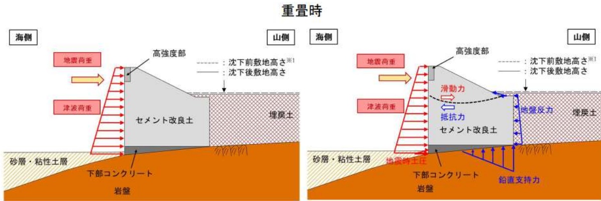
変形モード (防潮堤に生じる変位は小さい)
