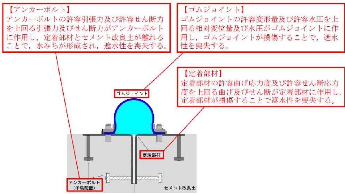
第 7-36 図 防潮堤(標準部)における止水ジョイントの構造上の弱部となる箇所(津波時及び重畳時)
