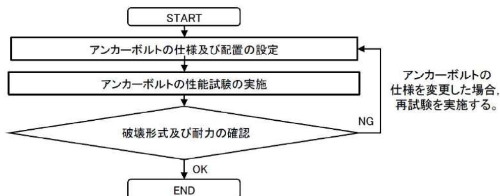
第 7-49 図 アンカーボルトの性能試験フロー
