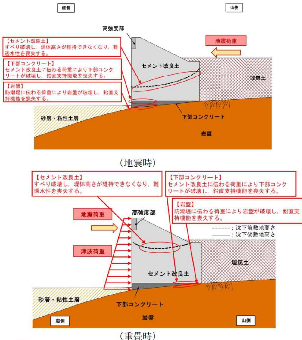
第 5-37 図 防潮堤（標準部）の構造上の弱部（地震時、重畳時）
