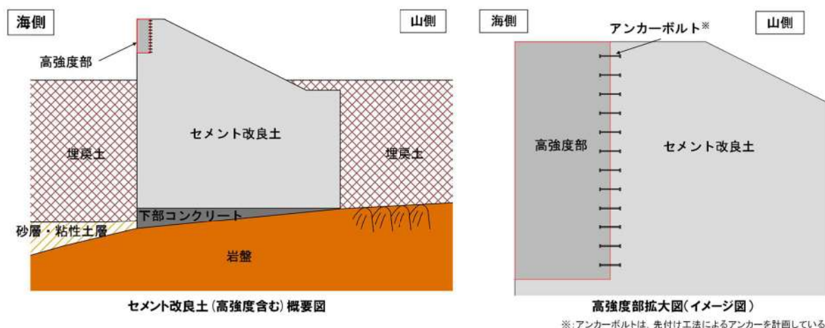
第 5-32 図 防潮堤（標準部）のセメント改良土及び高強度部の概略図
