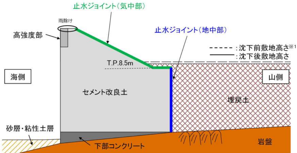
第 7-47 図 止水ジョイントの構造概要
