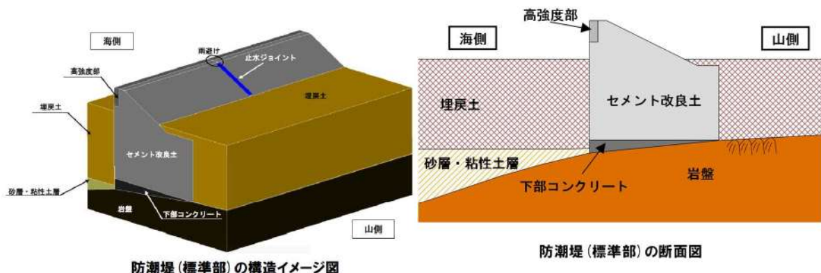
第 5-1 図 防潮堤（標準部）の構造概要
