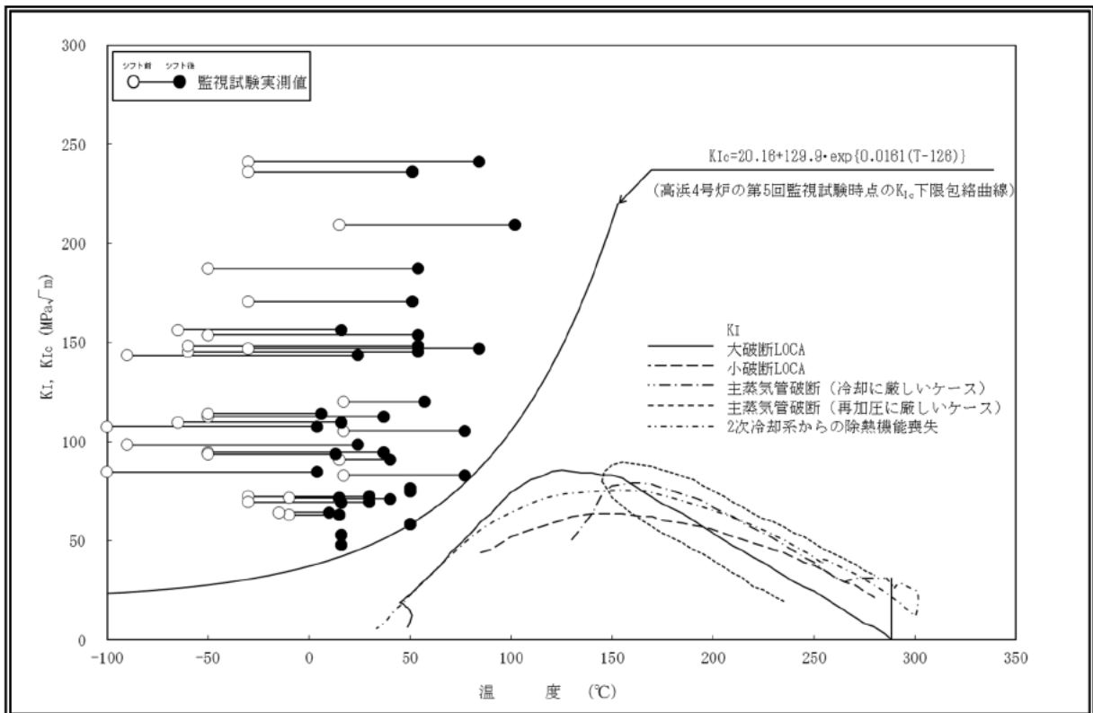
図 7 高浜 4 号炉 PTS 評価結果
