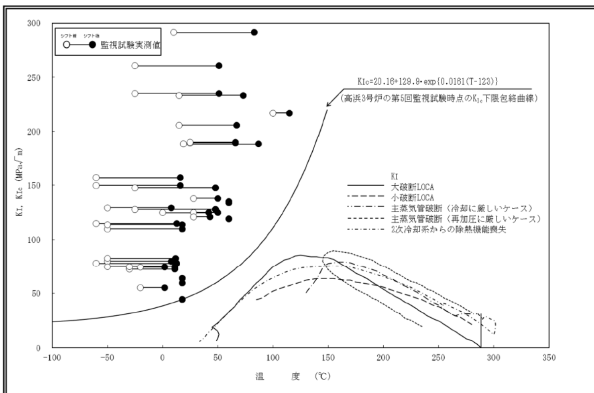
図7 高浜3号炉 PTS 評価結果
