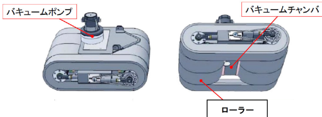
図 3. 5 点検装置 (壁面走行ロボット) 本体イメージ図
