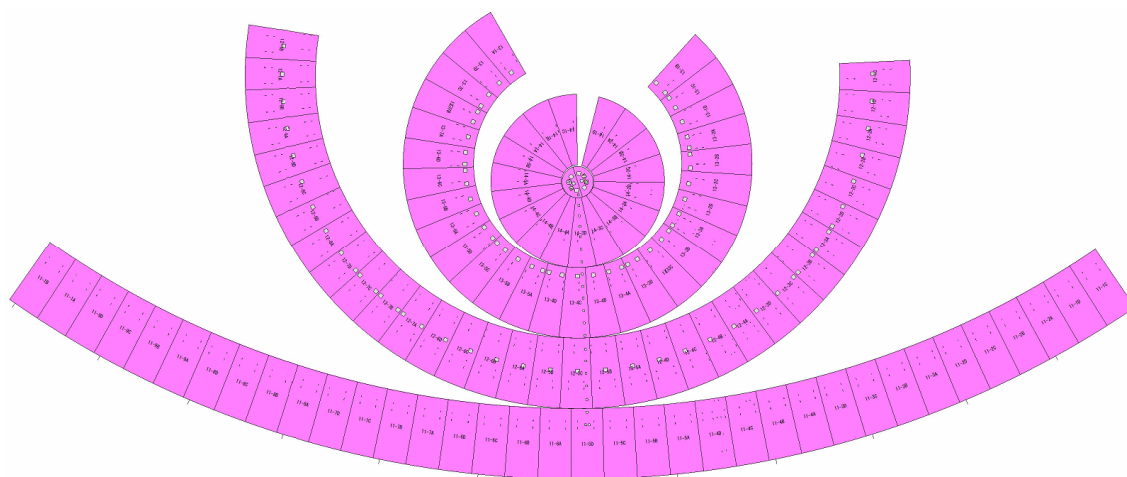
図3. 6 高浜4号炉 半球部外面
