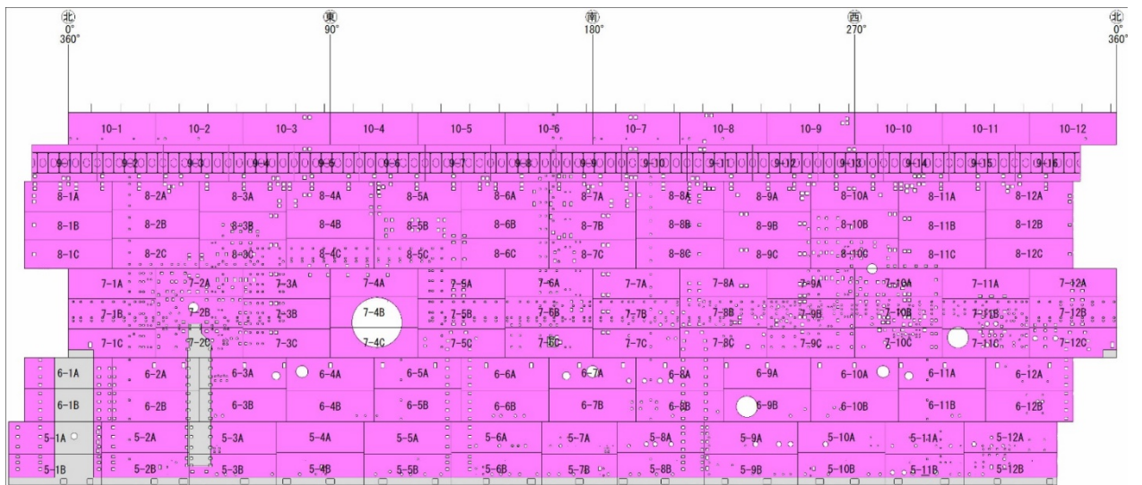
図3. 9 高浜4号炉 円筒部内面
