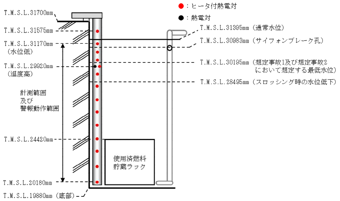
図1-6 使用済燃料貯蔵プール水位・温度 (SA広域) の設置図
