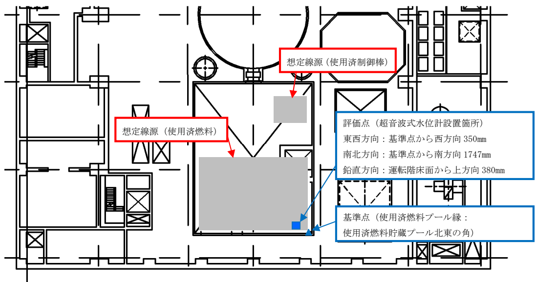
図4-9 使用済燃料貯蔵プール水位（超音波式）の評価点
