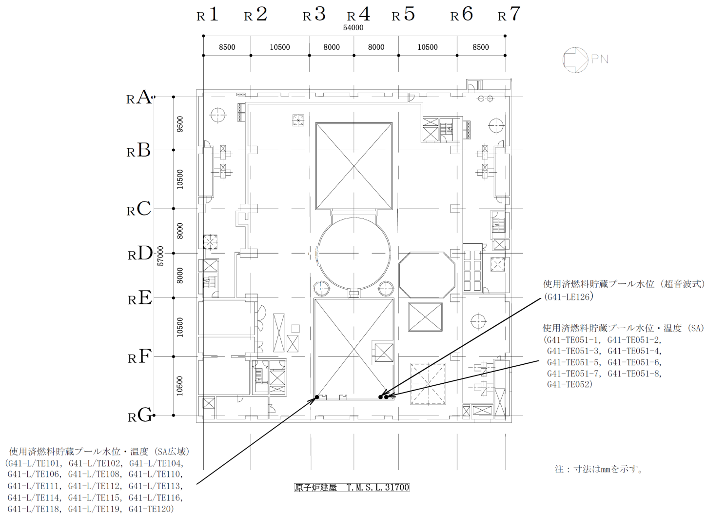
図 4-3 使用済燃料貯蔵プール水位（超音波式）の取付箇所を明示した図面
