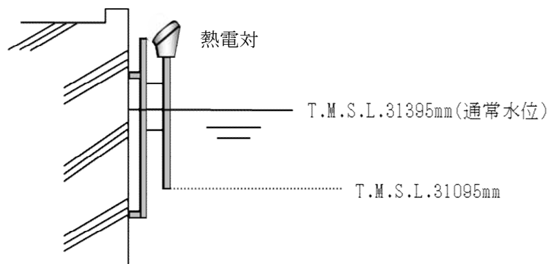
図1-1 使用済燃料貯蔵プール温度の設置図
