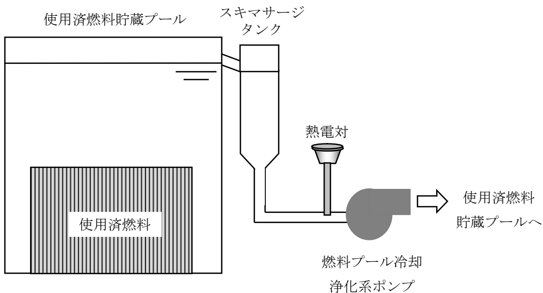
図1-2 燃料プール冷却浄化系ポンプ入口温度の設置図
