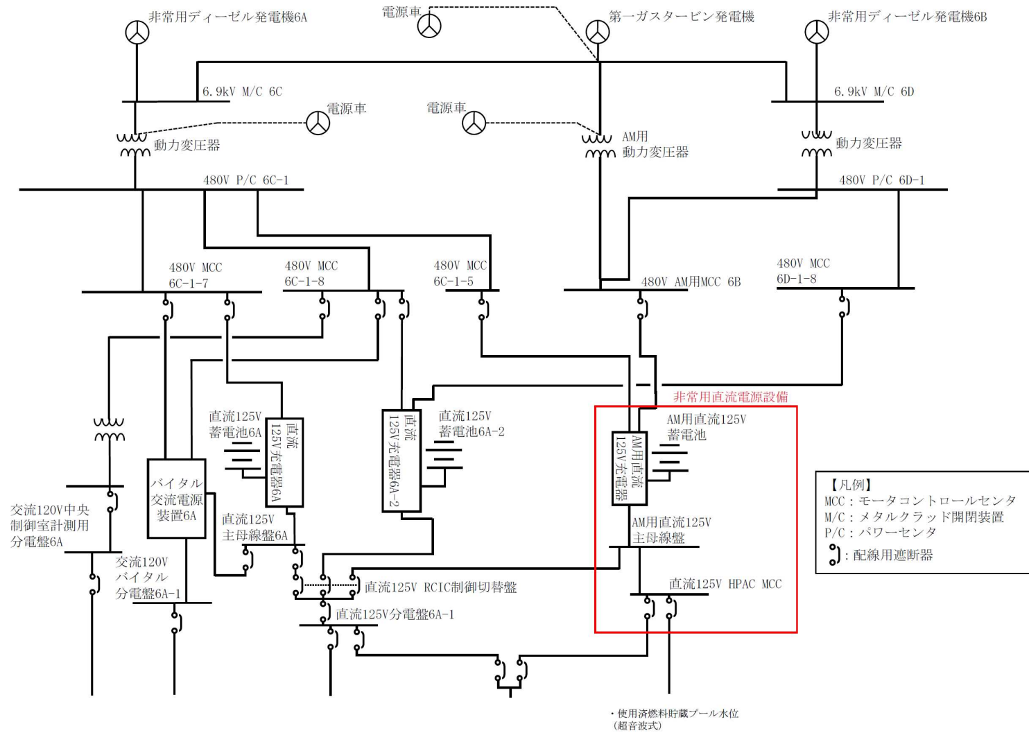
図 4-4 使用済燃料貯蔵プール水位 (超音波式) の概略電源系統図
