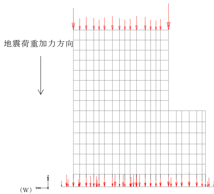
(a) 断面荷重図
