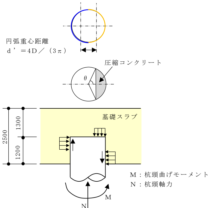
図 4-2 曲げモーメントの概要 (単位 : mm)
