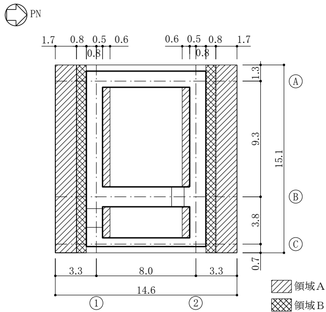
図 2-1 基礎スラブのせん断補強筋の配筋領域（単位：m）
