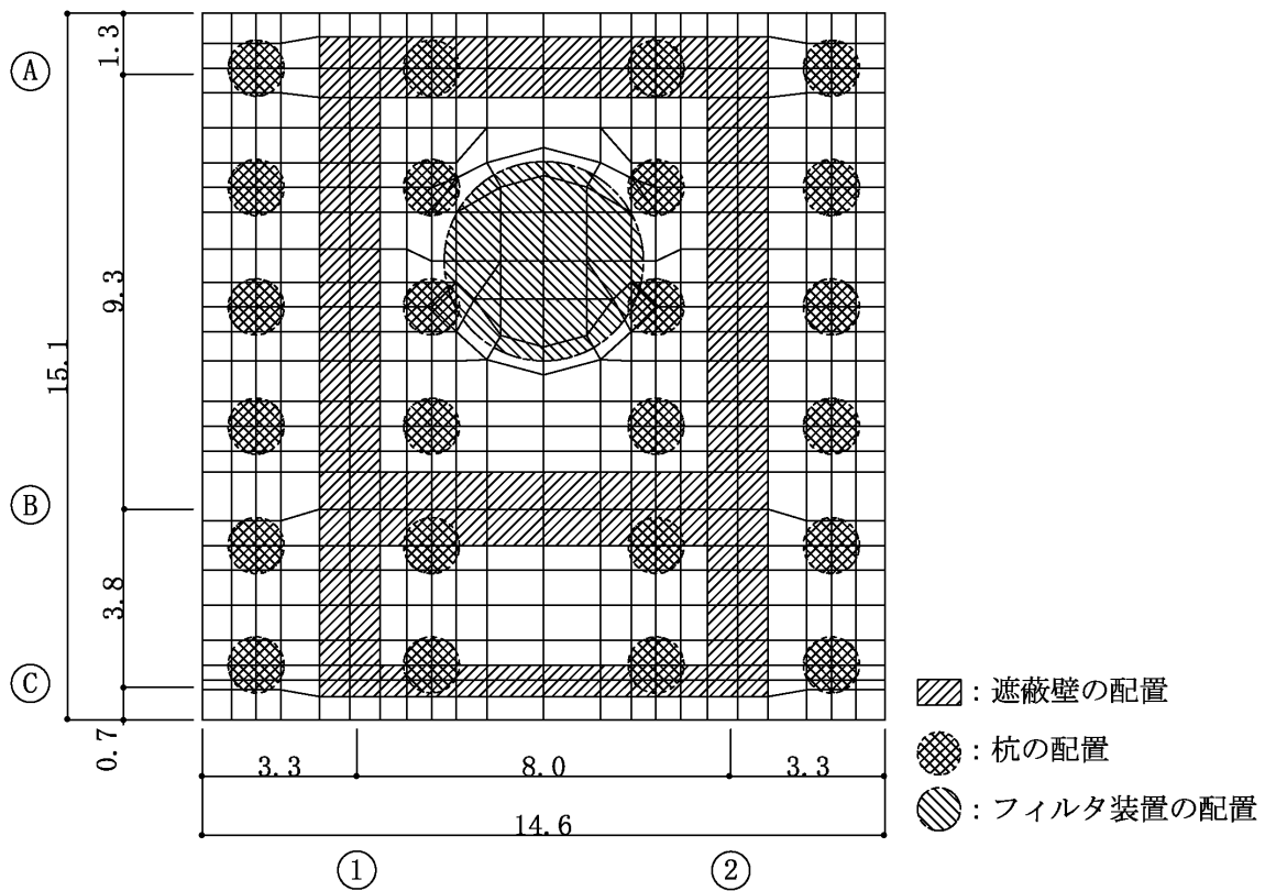
モデル概要（基礎スラブ）（単位：m）
