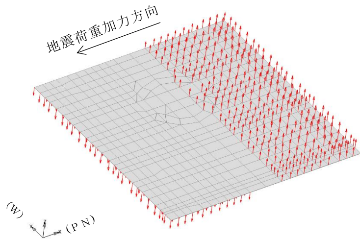
(b) 鳥瞰荷重図
