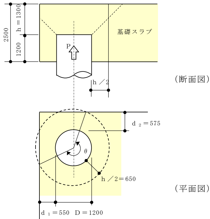
図2-1 杭の押抜きせん断の概要 (単位 : mm)
