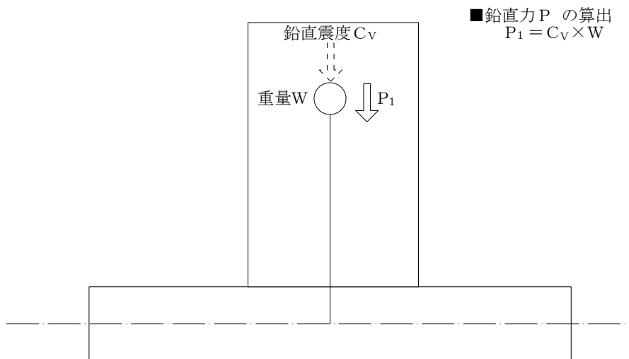
(a) 水平地震力
