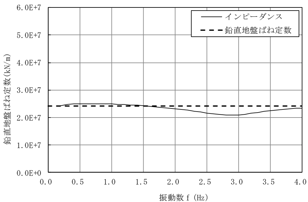
図 3-3 杭頭インピーダンス (鉛直方向)
