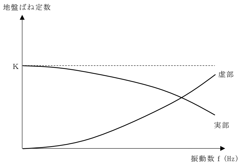
図 2-3 地盤ばね定数とインピーダンスの概念図
