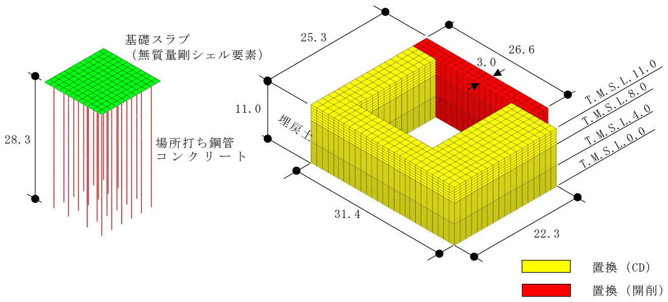
(a) 装置基礎－杭モデル
