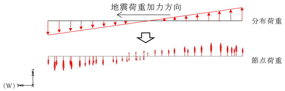
(a) 断面荷重図
