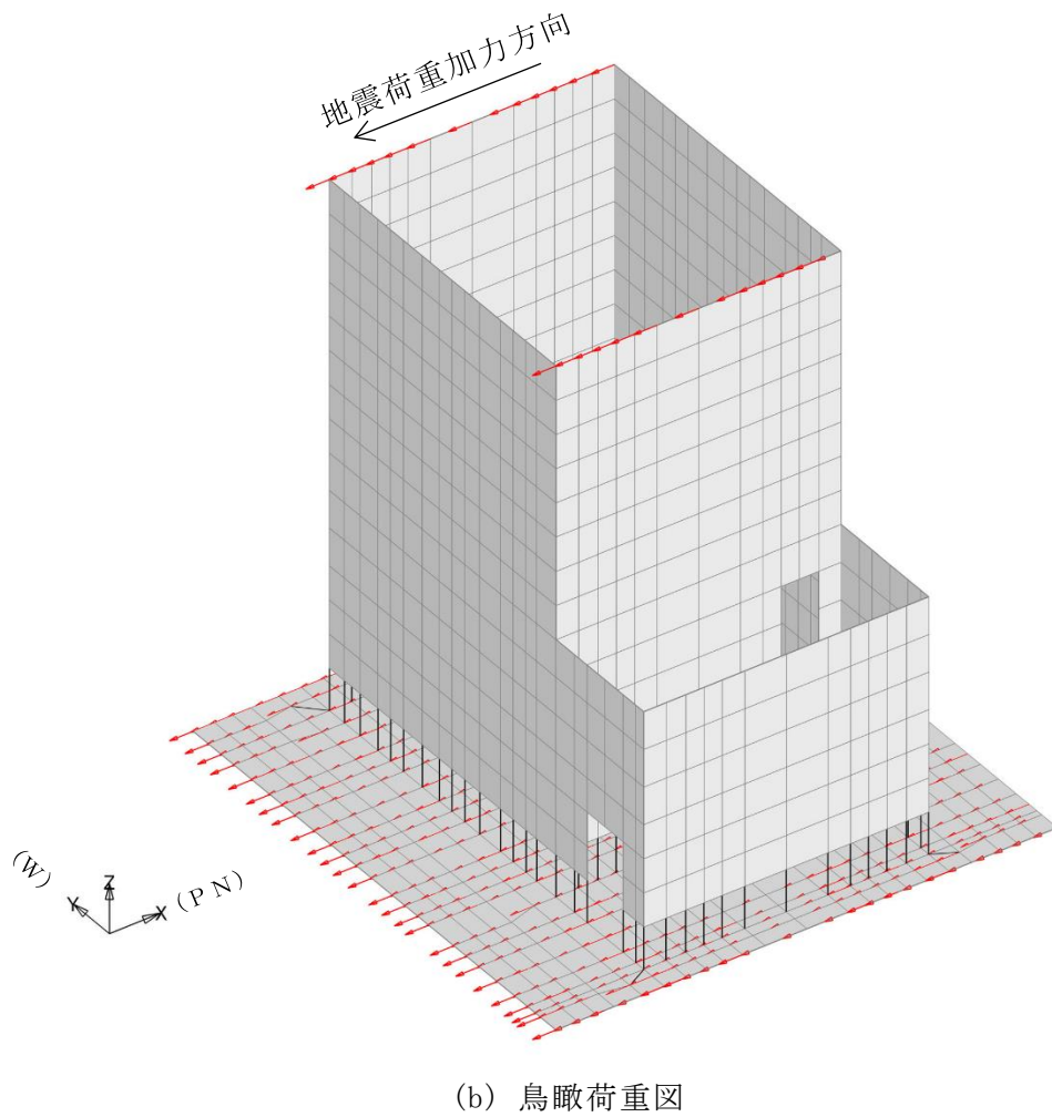
図 2-3 FEM モデルに入力する水平地震力 (NS 方向)
