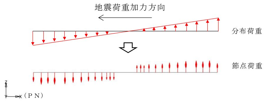
(a) 断面荷重図
