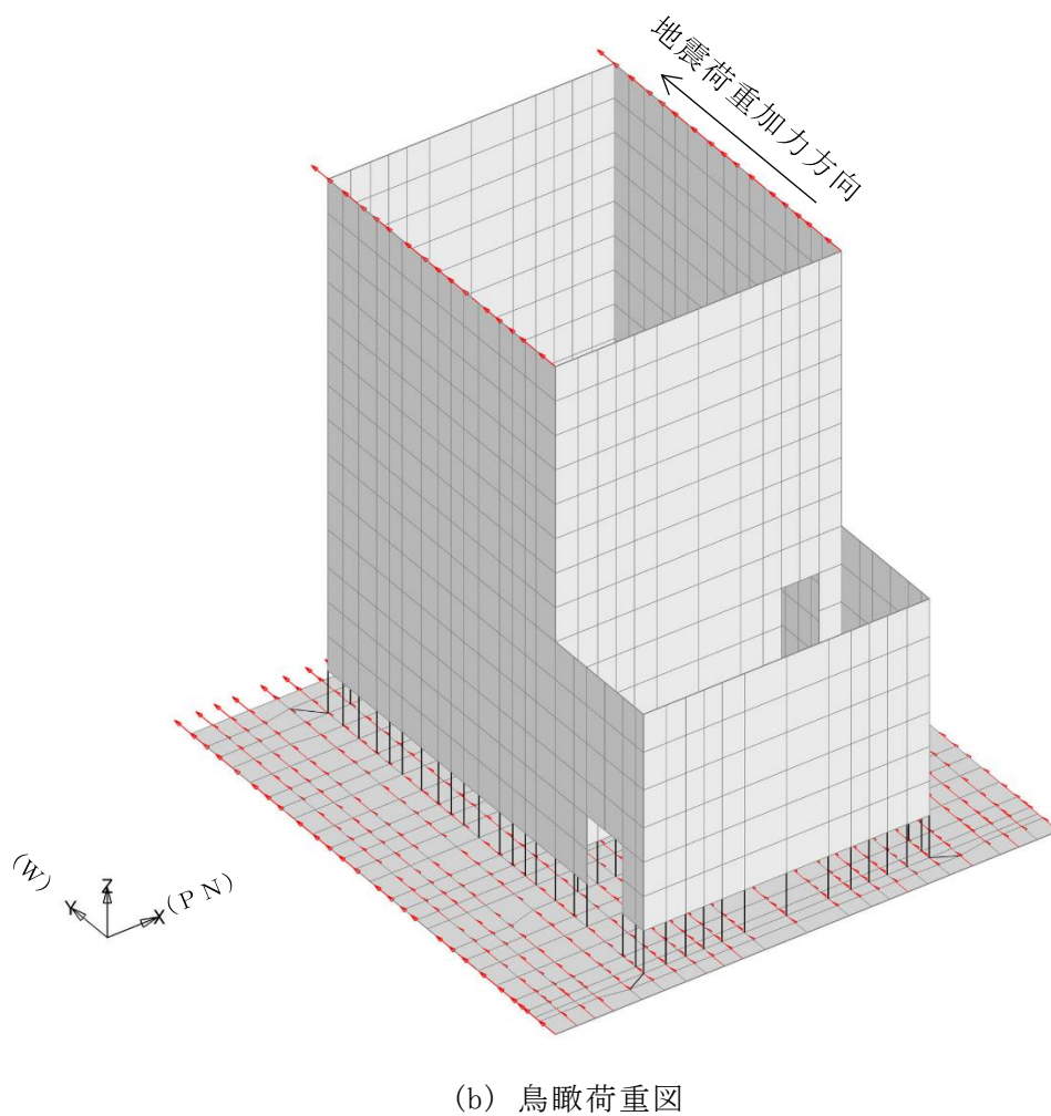
図 2-4 FEM モデルに入力する水平地震力 (EW 方向)
