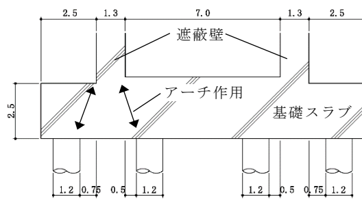
図 2-2 面外せん断力評価対象外範囲 (単位: m)
