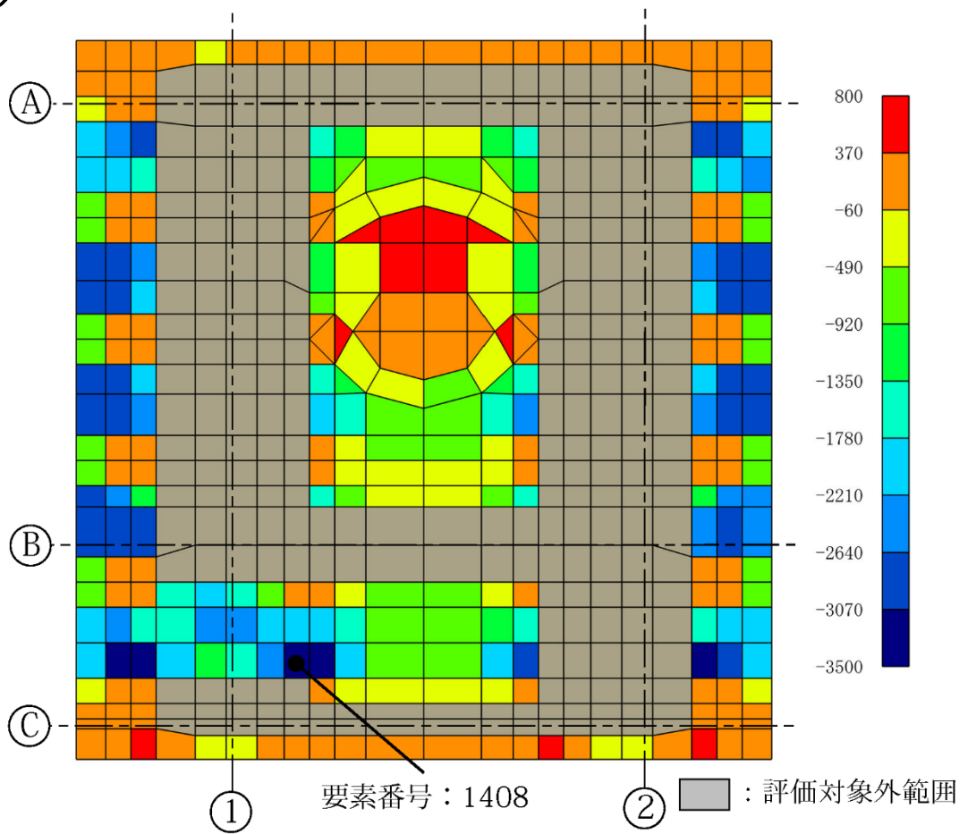
面外せん断力 (EW 方向, ケース 18)
