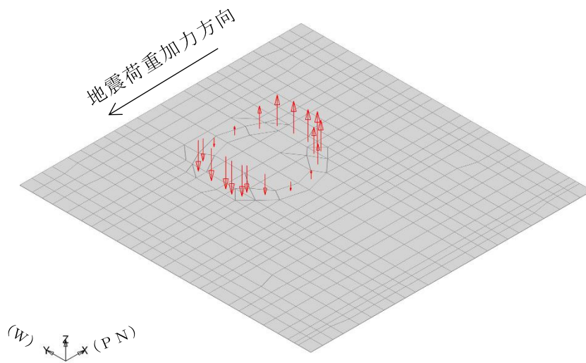
(b) 鳥瞰荷重図
