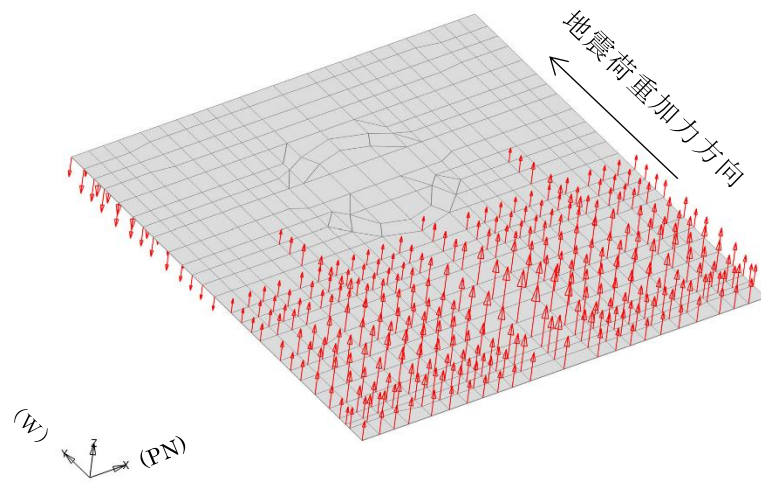
(b) 鳥瞰荷重図
