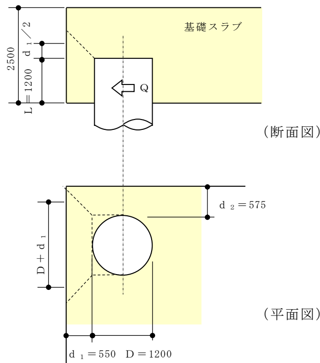
図4-1 杭の水平押抜きせん断の概要 (単位 : mm)
