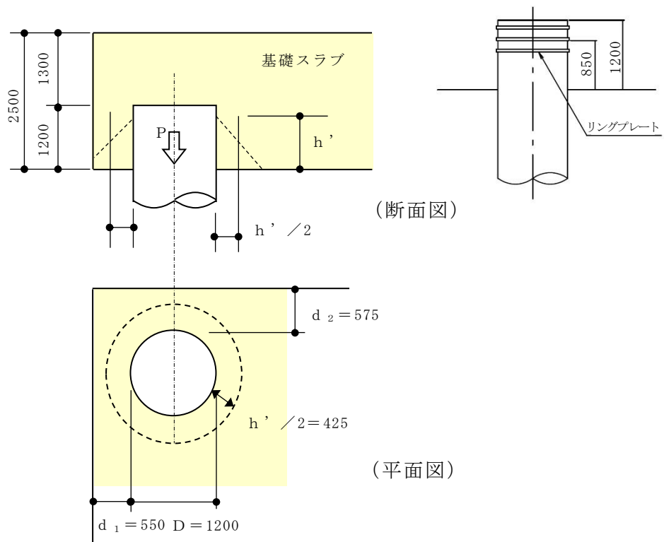
図3-1 杭の引抜きせん断の概要 (単位: mm)
