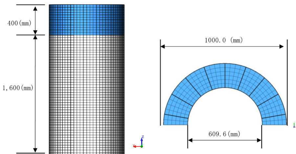
図 1 鋼コンクリート合成構造製の基礎構造物の三次元有限要素法解析モデル
