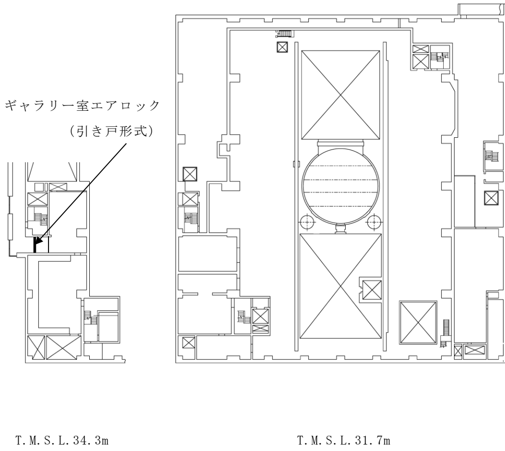
図 2-1 設置位置図 (2/2)
