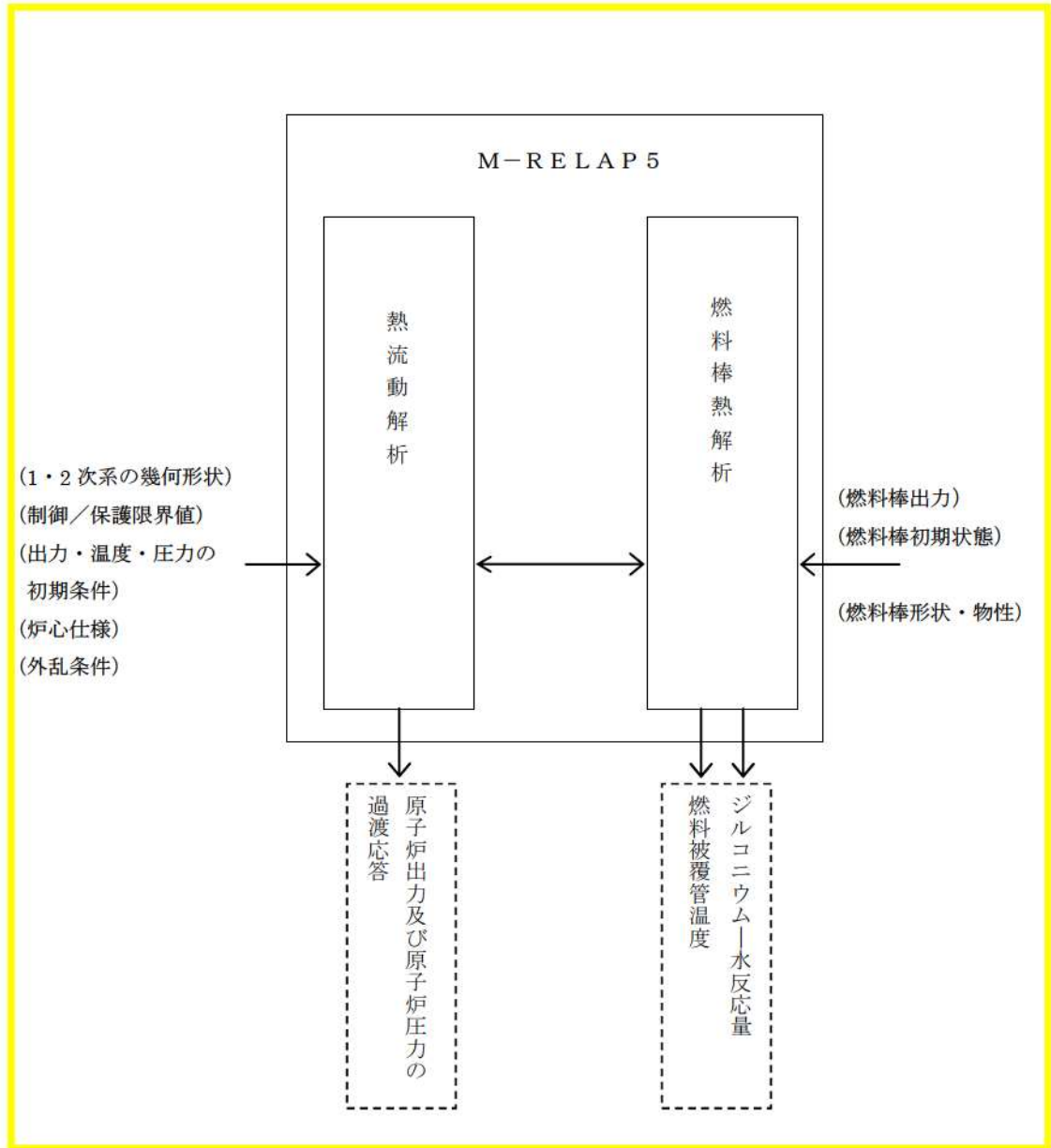
図 3-12 M-RELAP5 コードの入出力
