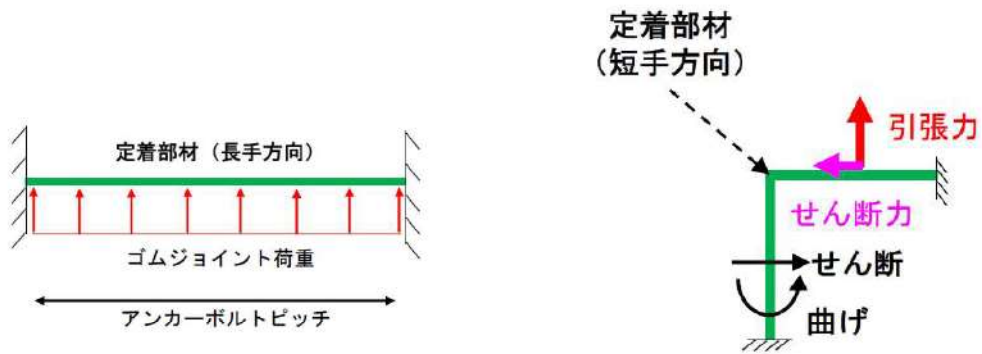
定着部材長手方向のモデル 定着部材短手方向のモデル 第 7-20 図 ゴムジョイントの張力による荷重とモデル化範囲のイメージ図 (解析②)
