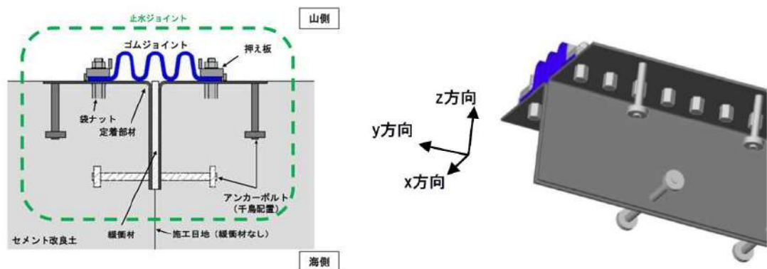
第 7-8 図 アンカーボルトの配置イメージ図
