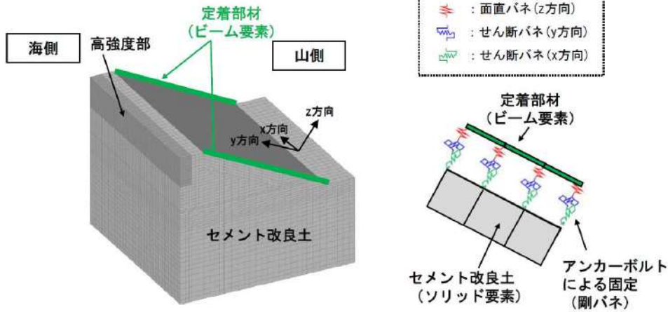
第 7-19 図 3次元静的FEM解析による解析モデルのイメージ図 (津波時の解析①)
