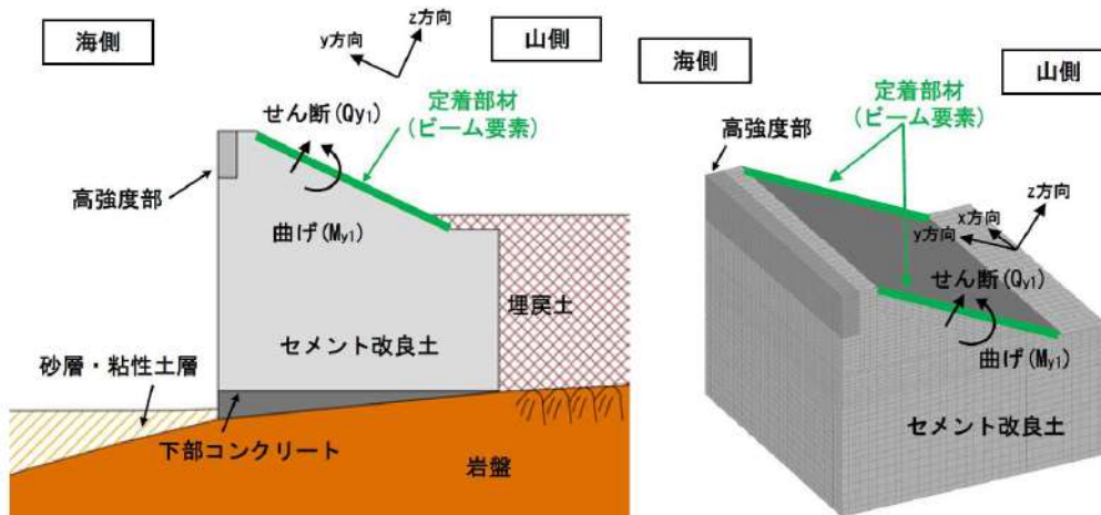
第 7-21 図 解析①のモデルと曲げ及びせん断のイメージ図 (左：地震時及び重畳時，右：津波時)
