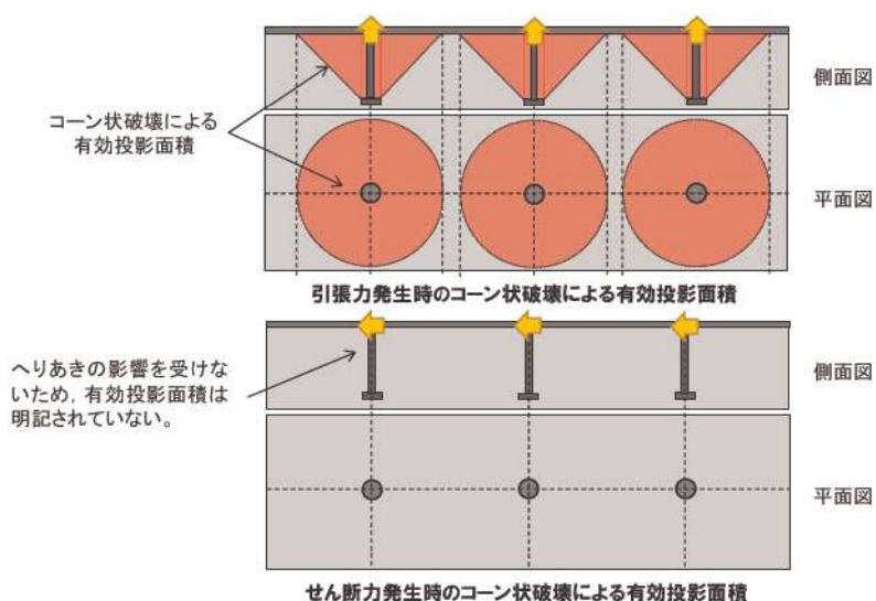
第 7-32 図 「各種合成構造設計指針」におけるアンカーボルトのコーン状破壊による有効投影面積
