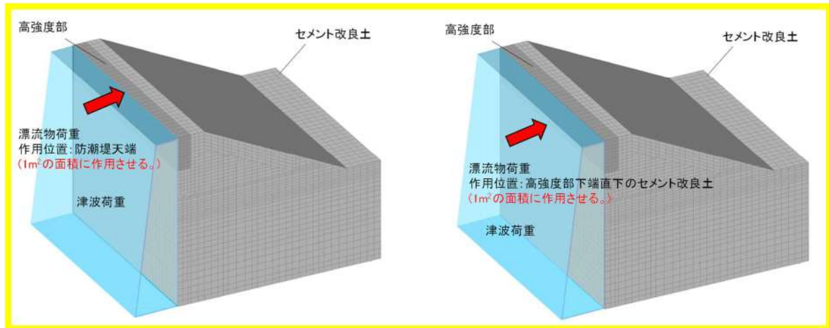
第 5-29 図 3次元静的FEM解析 解析モデル図（津波時）
