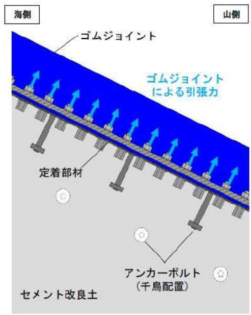
第 7-14 図 津波時にゴムジョイントの張力及び慣性力により定着部材及びアンカーボルトに生じる外力
