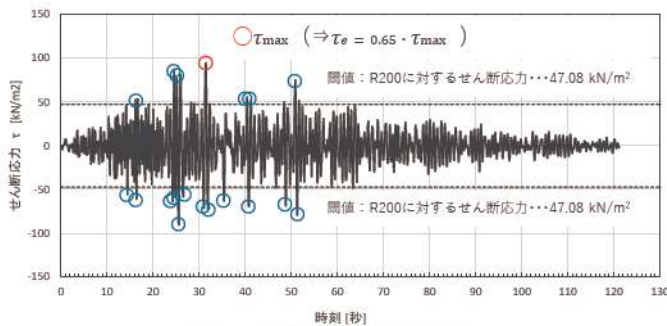
(例) 一次元地震応答解析結果
