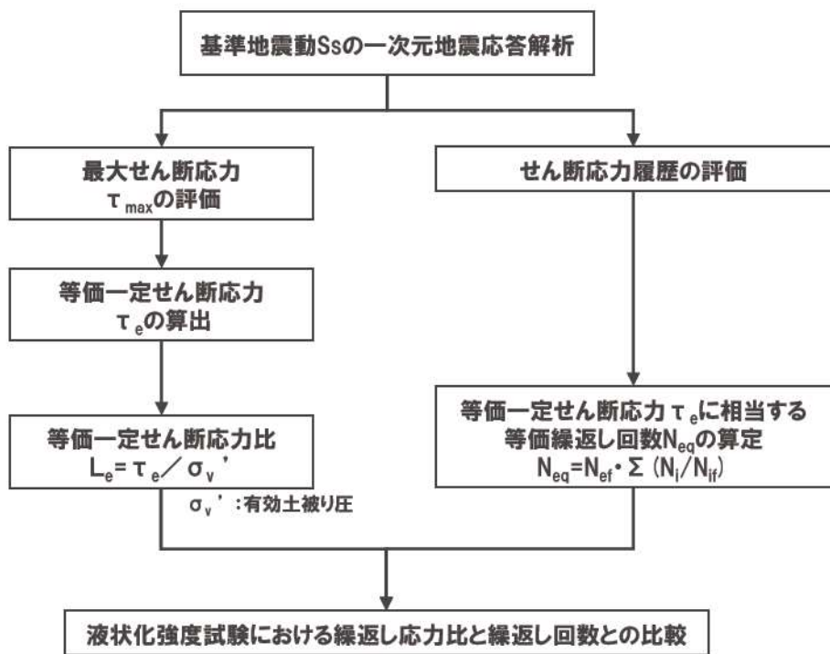
液状化強度試験の妥当性評価フロー
