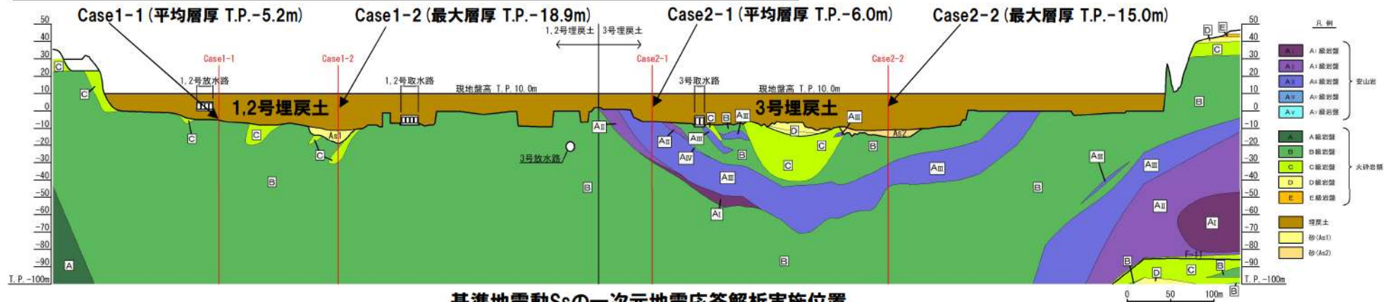
基準地震動Ssの一次元地震応答解析実施位置
