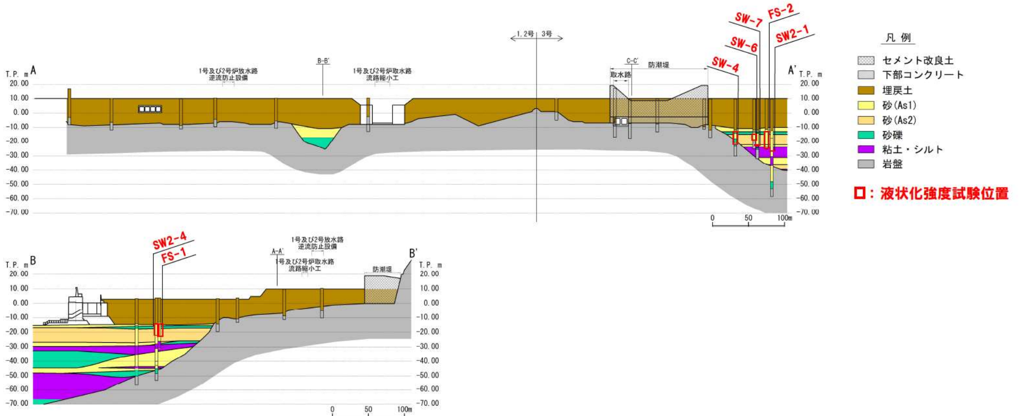
液状化強度試験位置図 (砂層)
