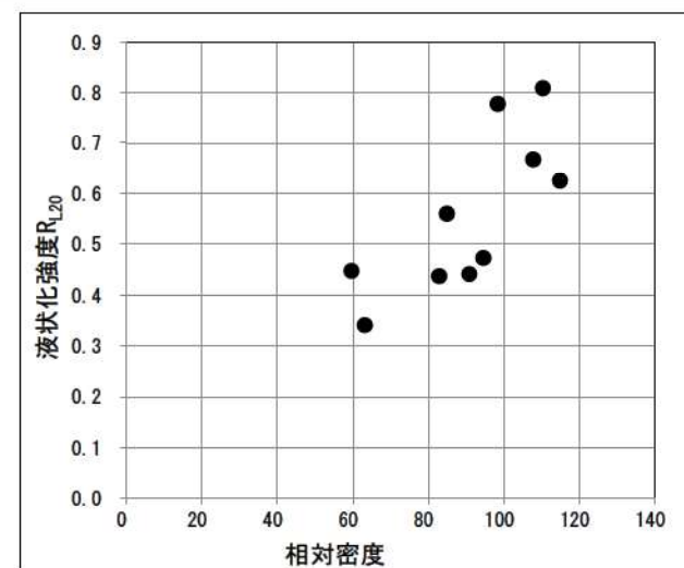
相対密度と液状化強度 R_{L20} の関係図(イメージ)
