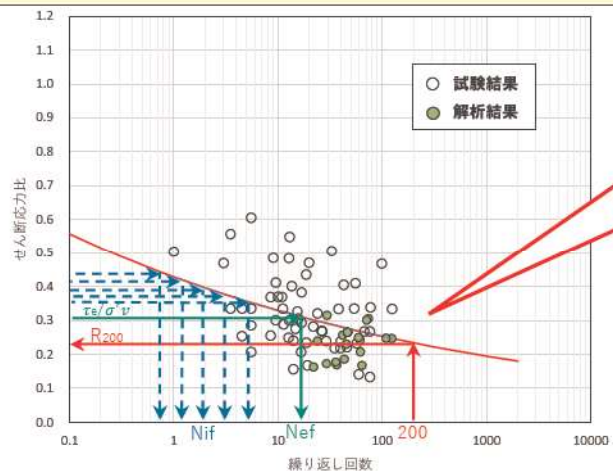
(例) 液状化強度試験結果と解析結果の比較
