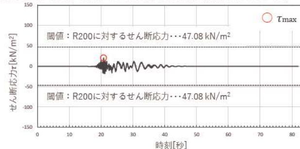
(例) せん断応力時刻歴 (Ss2-1-EW)
