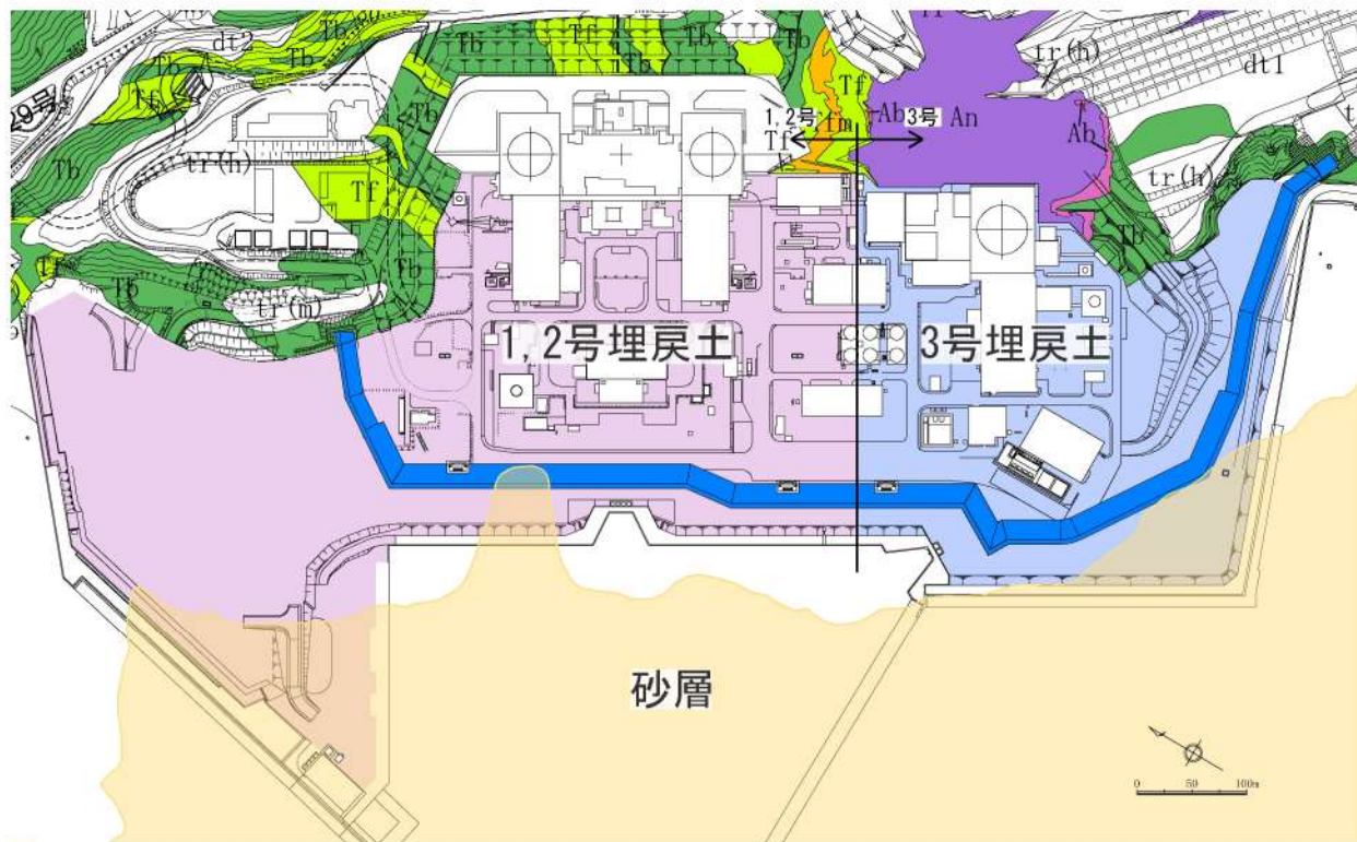
地質平面図
