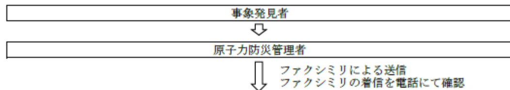
別図第3 原子力災害対策特別措置法第10条第1項に基づく通報体制 (1/2) (1) 社内での事象発生時の通報体制
