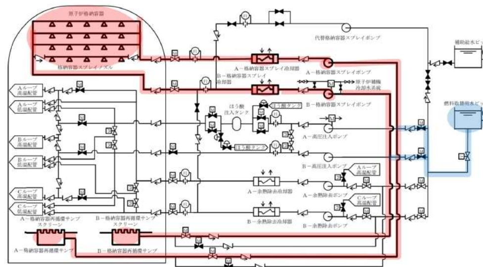
泊3号炉 格納容器スプレイ及び格納容器スプレイ再循環
