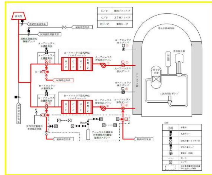
図 53-4-1 アニュラス空気浄化設備による水素排出 (交流動力電源及び直流電源が健全である場合)
