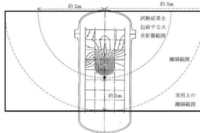
図6 イグナイタによる火炎影響範囲と分離範囲の設定 (イグナイタ設置工事において設定)
