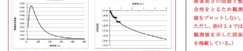
第 2.3.5.3 図 被害幅の確率密度分布
