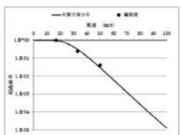
図 1.3.13 風速の超過確率
