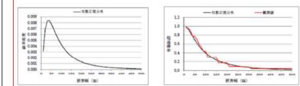
図 1.3.14 被害幅の確率密度分布
