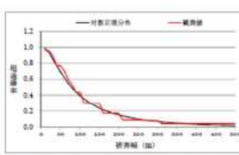
図 1.3.15 被害幅の超過確率
