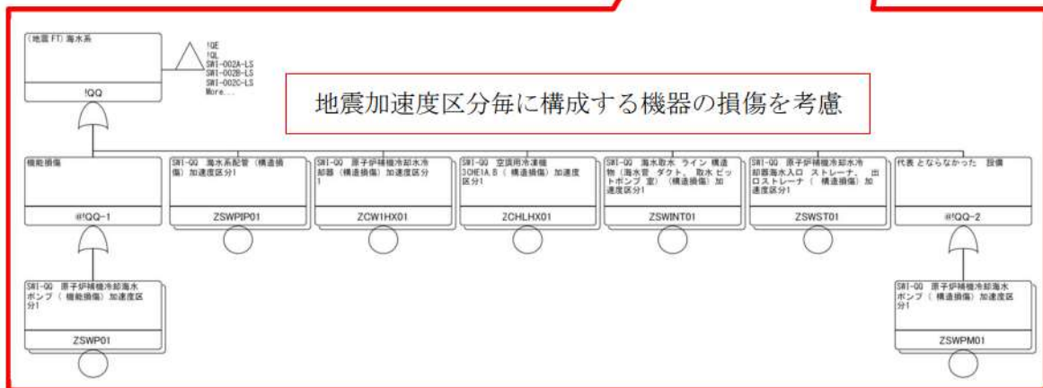
(緩和設備の地震による直接的な損傷の代表例「海水系フォールトツリー」)
