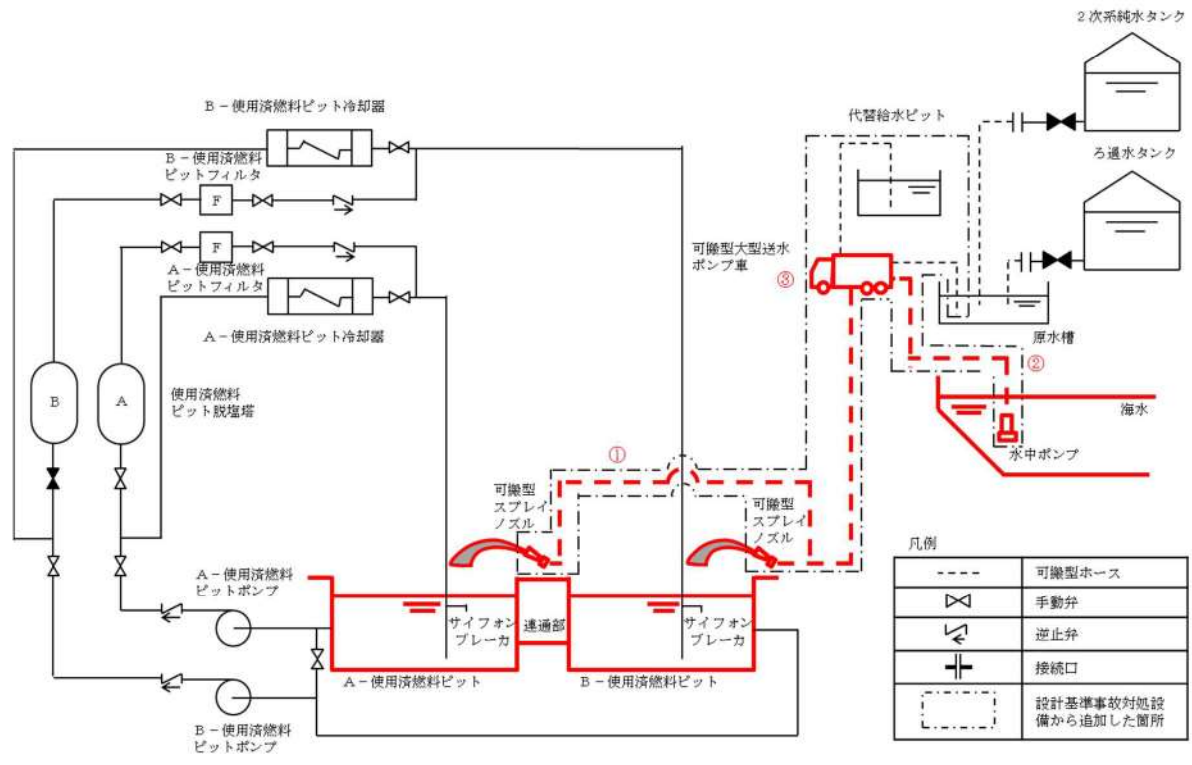
図 54-4-2 使用済燃料ピットへのスプレィ
