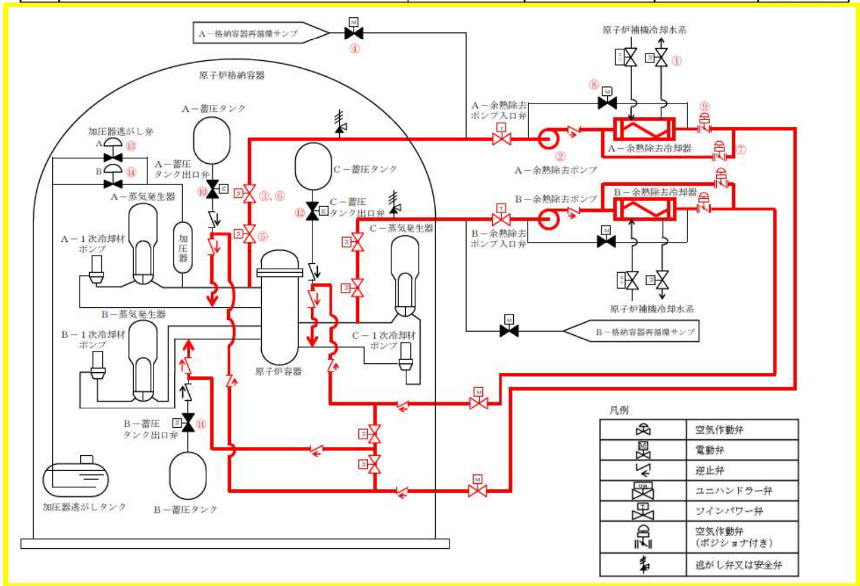
図 45-4-3 1次冷却系のフィードアンドブリード（余熱除去設備による冷却）
