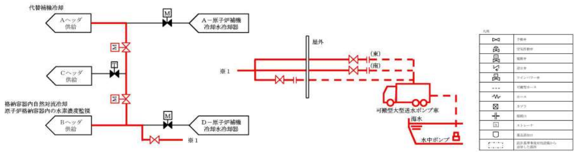
図 2.13-5 海を水源とした場合に用いる設備（格納容器内自然対流冷却，代替補機冷却及び原子炉格納容器内の水素濃度監視）
