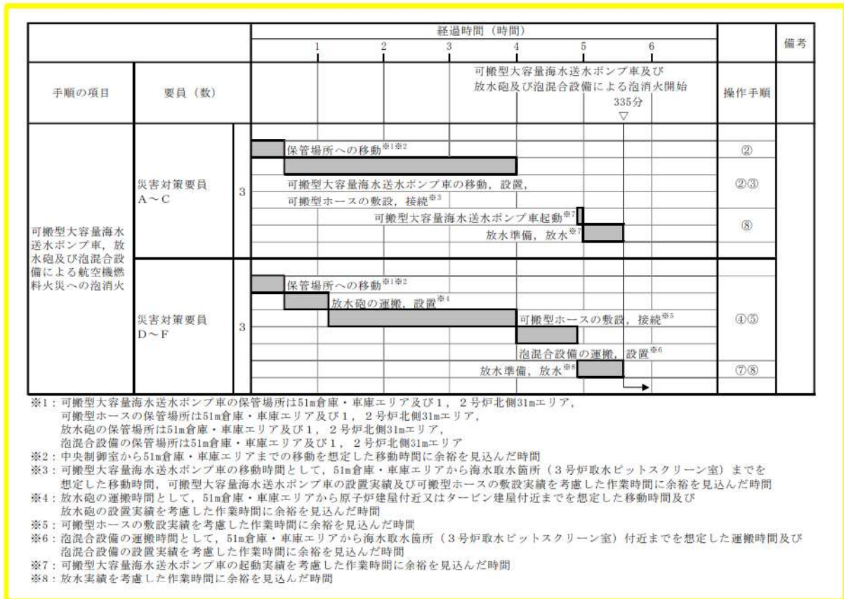
図2.12-8 可搬型大容量海水送水ポンプ車、放水砲及び泡混合設備による泡消火 タイムチャート※
