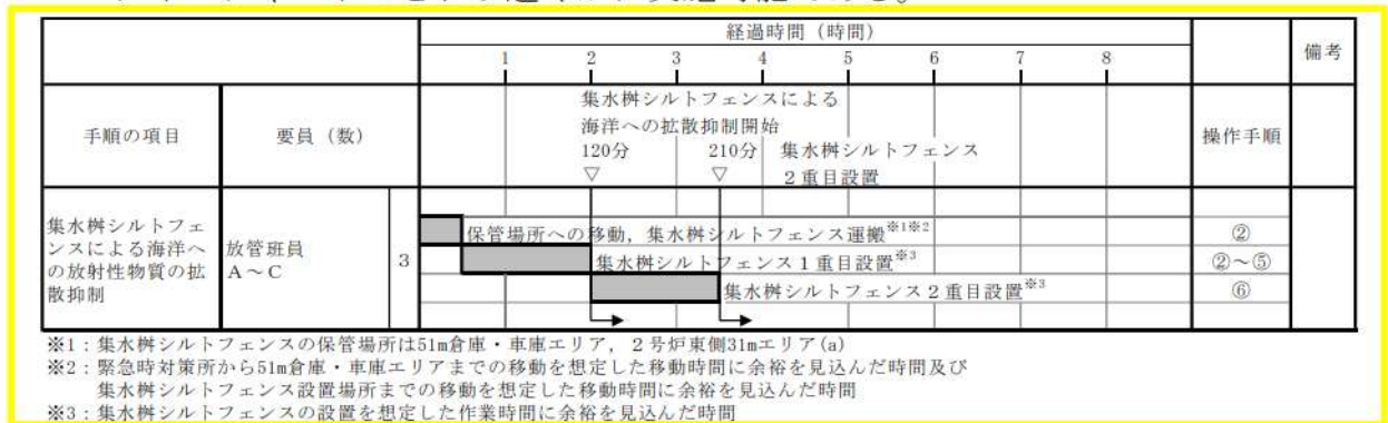
図2.12-4 海洋への拡散抑制設備（シルトフェンス）による海洋への放射性物質の拡散抑制タイムチャート ※1
