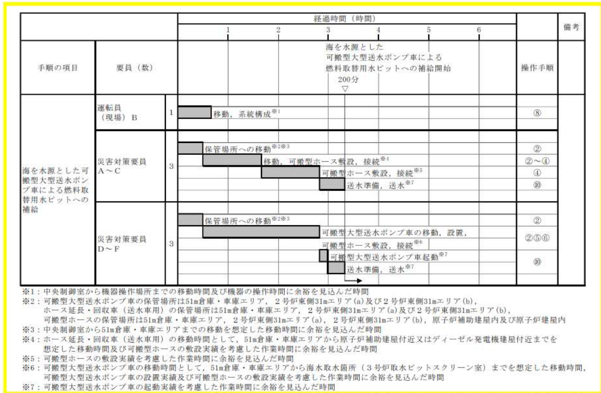
図2.13-15 海を水源とした可搬型大型送水ポンプ車による燃料取替用水ピットへの補給 タイムチャート
