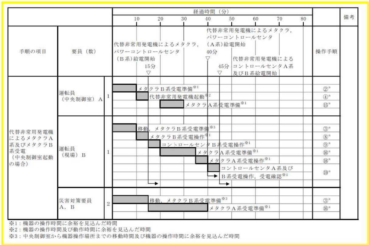
図 2.14.15 代替非常用発電機による非常用高圧母線 (6-A) 及び非常用高圧母線 (6-B) 受電のタイムチャート*
