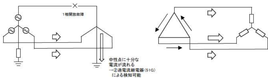
第 2. 2. 1. 14 図 地絡過電流継電器 (51G) による検知 (イメージ) (主変圧器)
