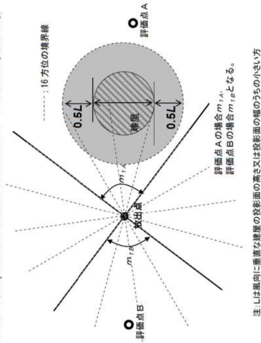
注: Lは風向に垂直な建屋の投影面の高さ又は投影面の幅のうちの小さい方 図 5.5 建屋の風下側で放射性物質が巻き込まれる風向の方位 m_1 の選定方法 (水平断面での位置関係)
