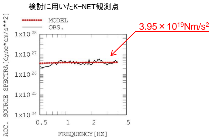
2011年7月10日三陸沖の地震の観測加速度スペクトルと \omega^{-2} モデルの比較 (短周期レベルの推定には4Hz以下を用いた)
