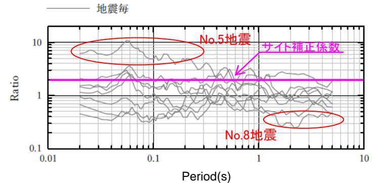
海洋プレート内地震のNoda et al.(2002)に対するサイト補正係数(本編資料p.132に一部加筆)
