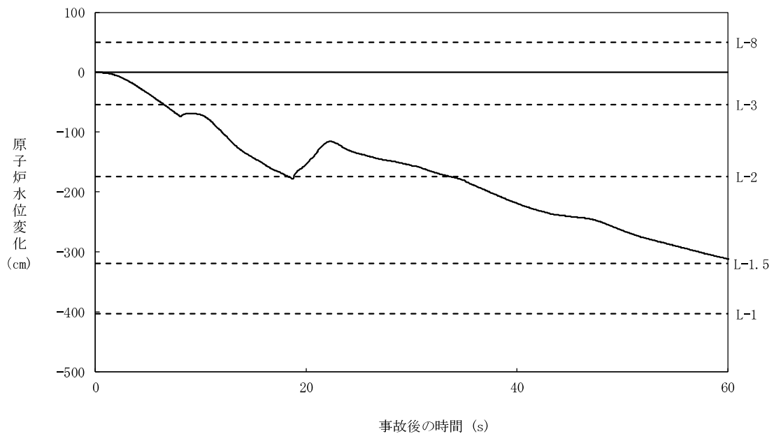
図 5.3.5-6 原子炉水位(シュラウド外水位)の時間変化（給水流量の全喪失+CCF）
