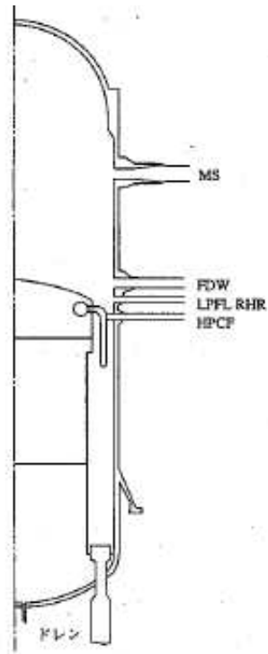
添付図 1-2 ABWR における RPV 接続主要配管の位置
