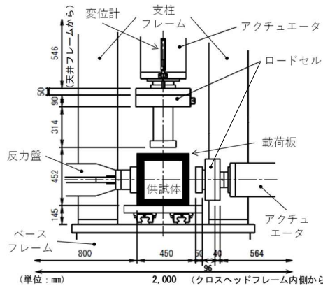
図-2 力学試験機部分の立面図 (供試体周辺の拡大)
