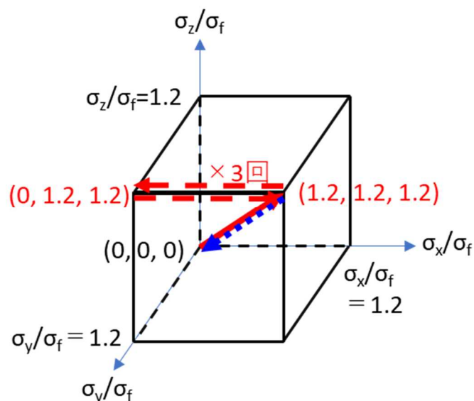
図2 応力履歴図
