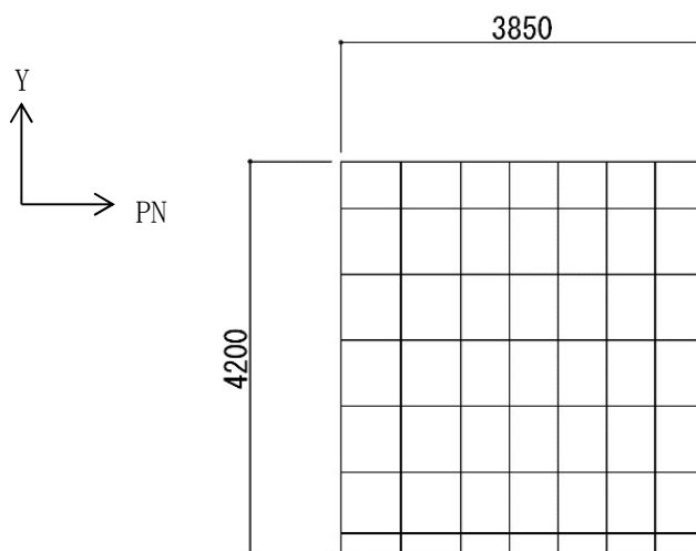
(e) 北妻壁
