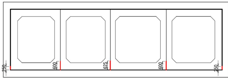
A-A断面
