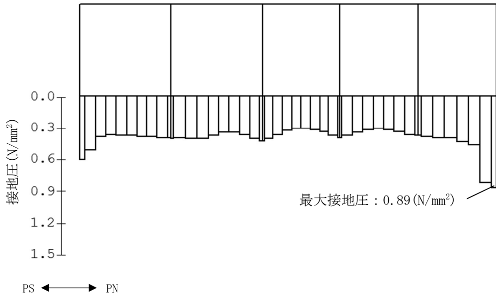
図 5-118 補機冷却用海水取水路（南側）の最大接地圧分布図 （解析ケース①，地震動 Ss-1--）
