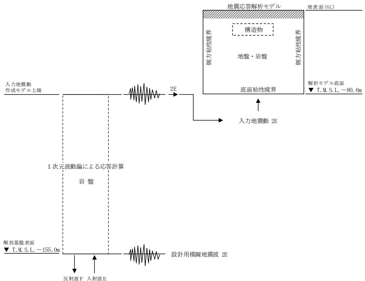
図 5-69 入力地震動算定の概念図
