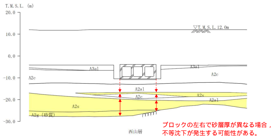
図 2 - 25 スクリーン室 (1BL) の断面図
