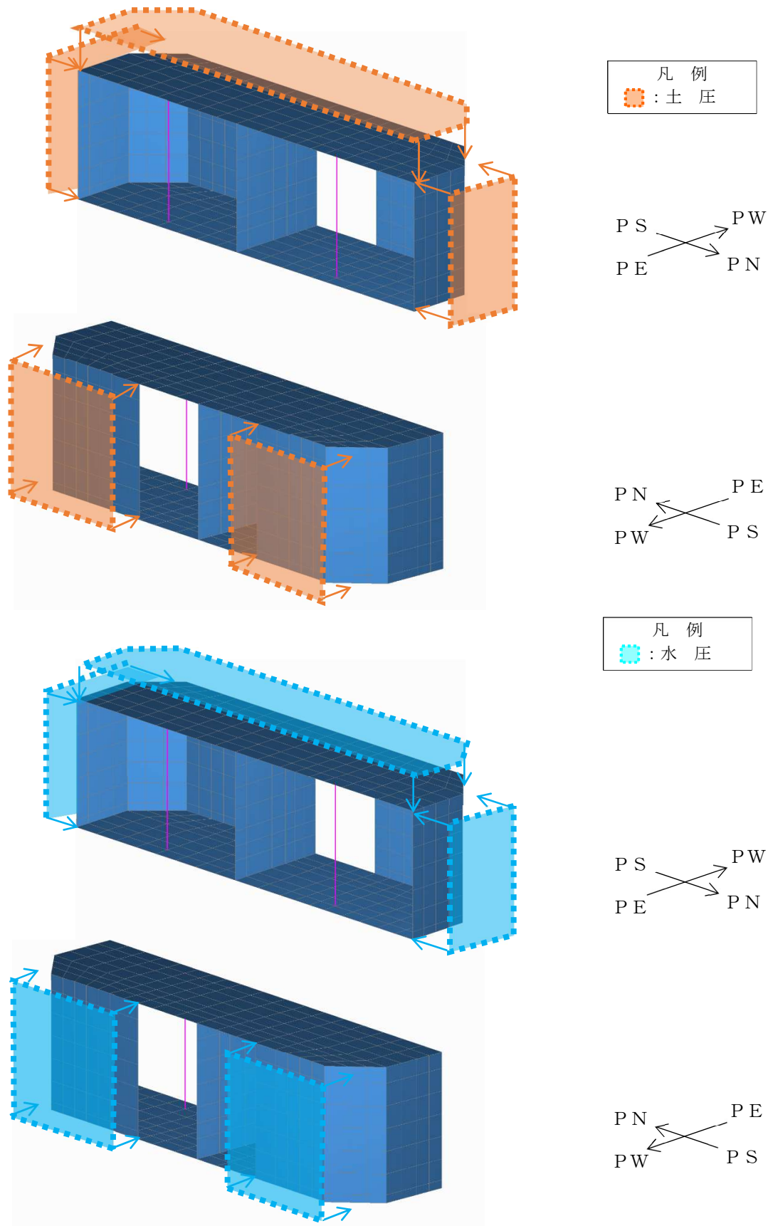
図 5-68 補機冷却用海水取水路（北側）の土圧及び水圧の概略図
