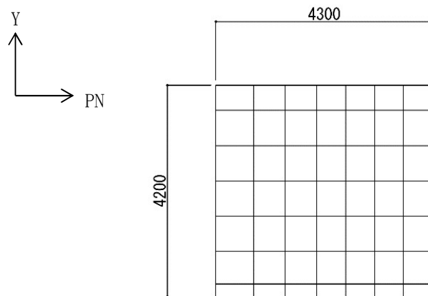
(e) 北妻壁
