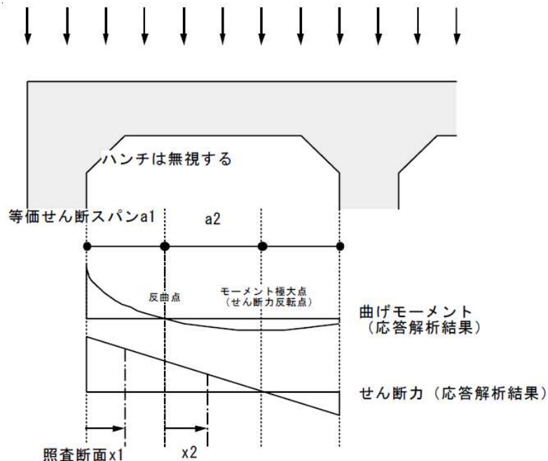
図 5-96 等価せん断スパンの設定方法
