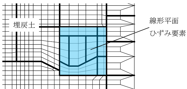
図 5-35 補機冷却用海水取水路（北側）の地震応答解析モデル（C-C断面，構造物拡大） (1/2)
