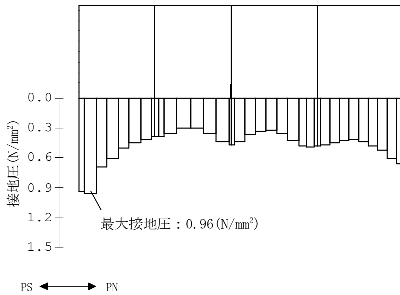
図 5-119 補機冷却用海水取水路（北側）の最大接地圧分布図 （解析ケース②，地震動 Ss-1+-）
