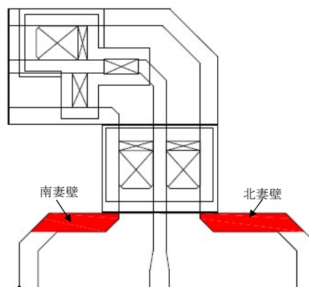
図 5-99 補機冷却用海水取水路（北側）の妻壁の位置
