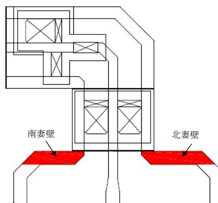
図 5-101 補機冷却用海水取水路（北側）の妻壁の位置
