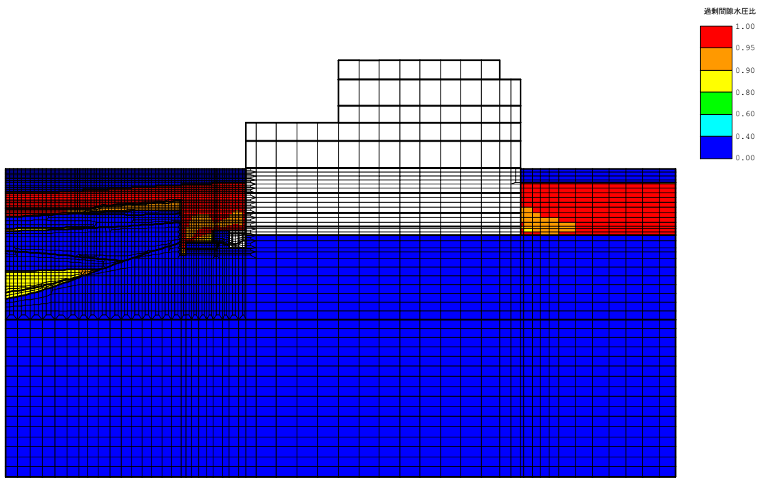
(a) 全体図
