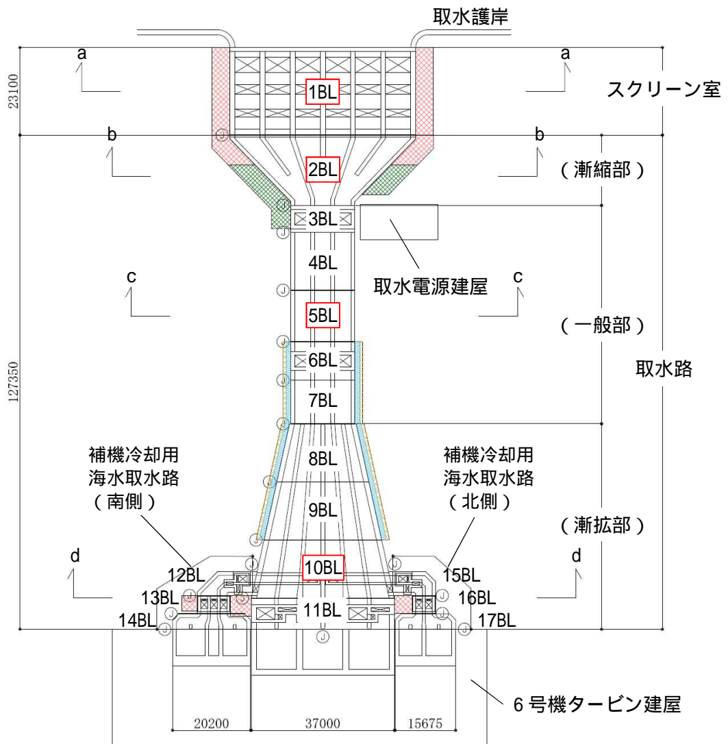
図 2 - 21 横断面方向の二次元地震応答解析実施位置
