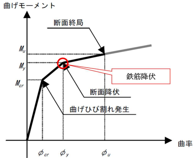
図 5-97 貯水機能を要求する鉄筋コンクリート部材の許容限界
