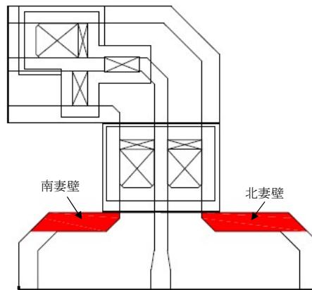
図 5-131 補機冷却用海水取水路（北側）の妻壁の位置
