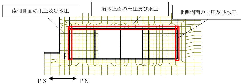
(A-A断面)
