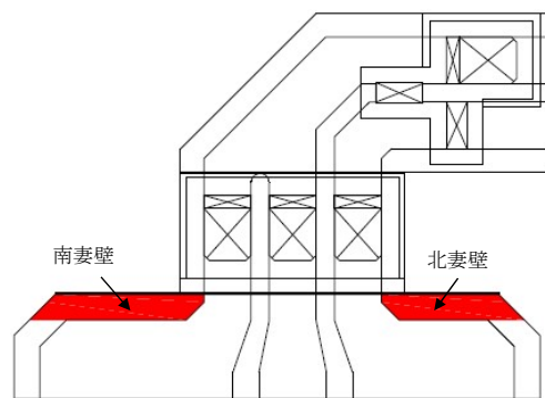
図 5-100 補機冷却用海水取水路（南側）の妻壁の位置
