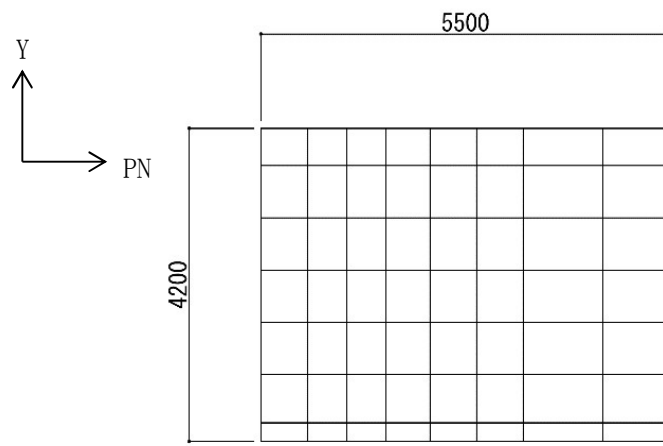
(d) 南妻壁
