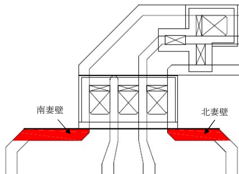
図5-130 補機冷却用海水取水路(南側)の評価位置
