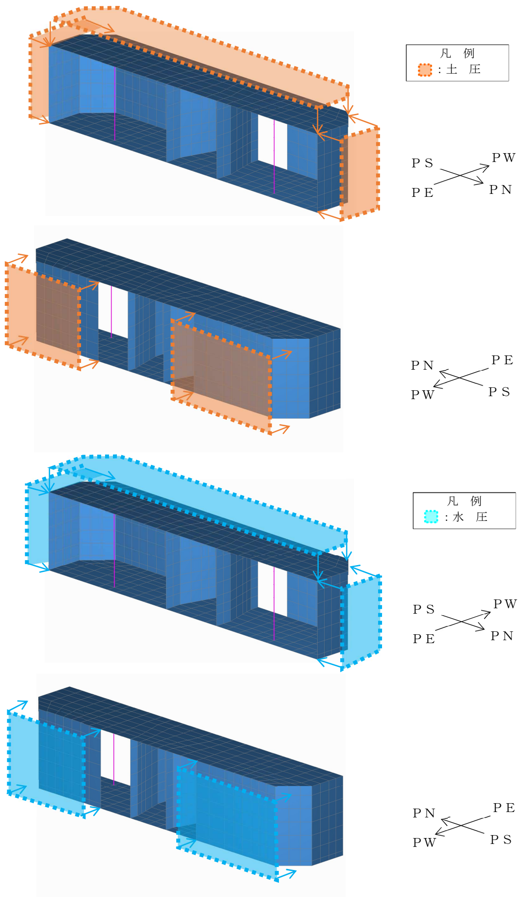
図 5-67 補機冷却用海水取水路（南側）の土圧及び水圧の概略図
