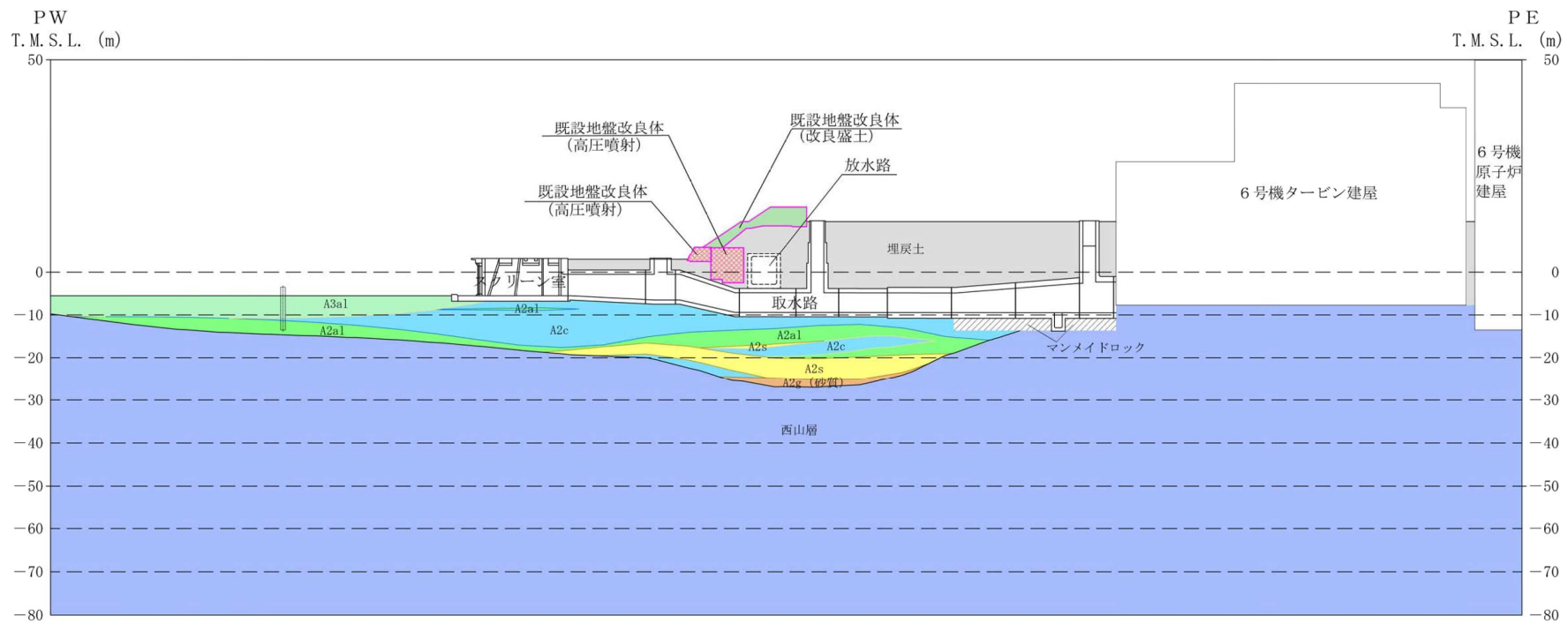
図 2-3 スクリーン室及び取水路の縦断方向の地質断面図
