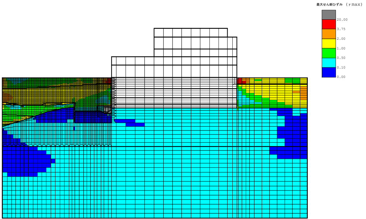
(a) 全体図
