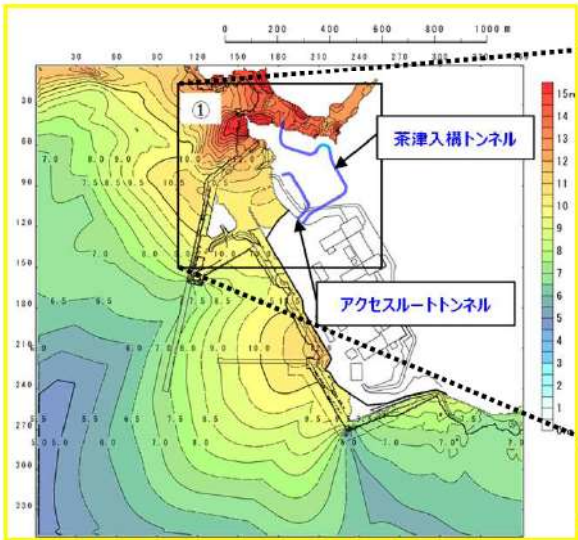
最大水位上昇量分布図※1 (基準津波は今後変更となる可能性あり)
