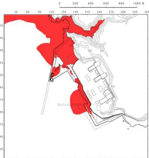
地山斜面(茶津側)で水位が大きくなる波源 (波源J・北及び南防波堤損傷)
