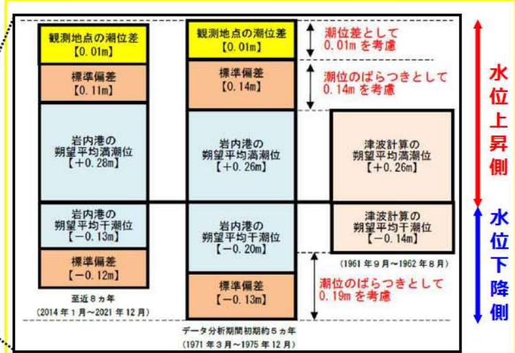
潮位変動の概念図
