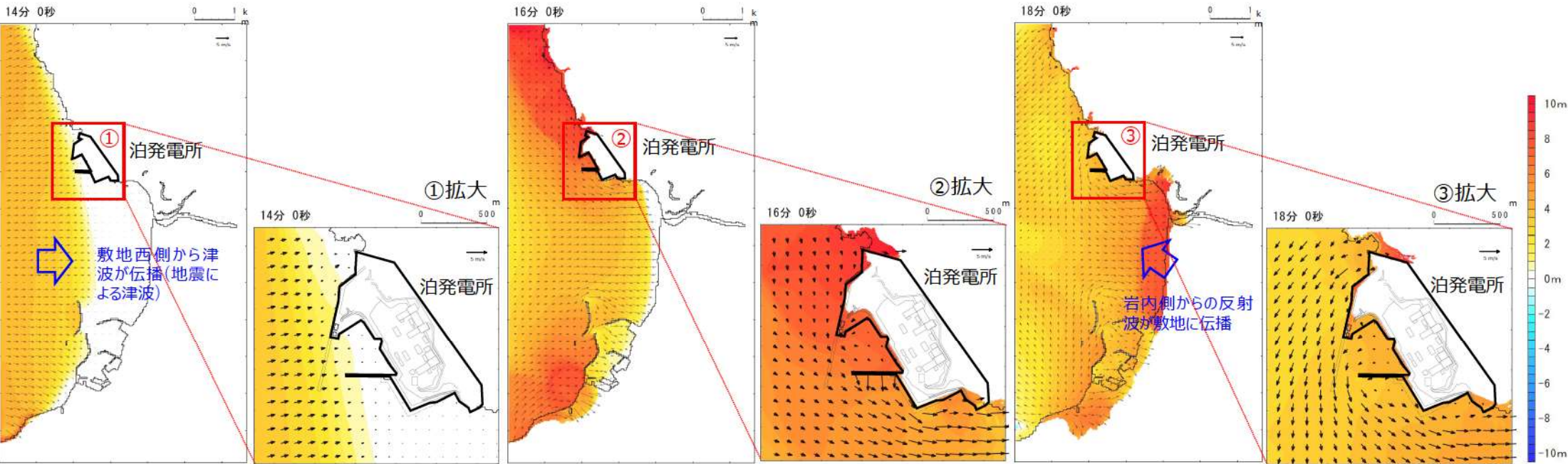
水位・流速分布の経時変化(スナップショット)(1/2)※
