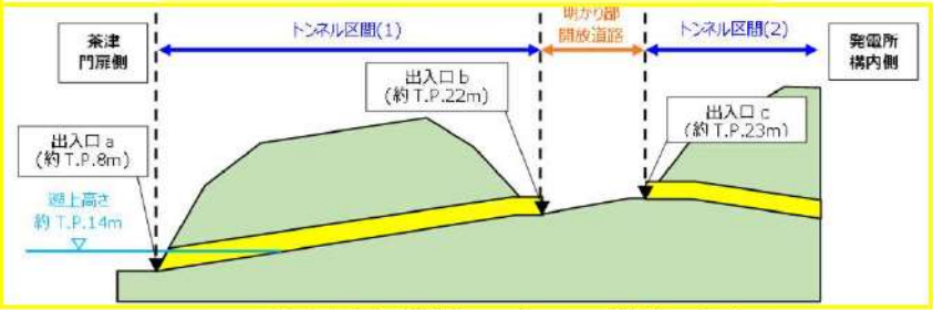
茶津入構トンネル 断面図
