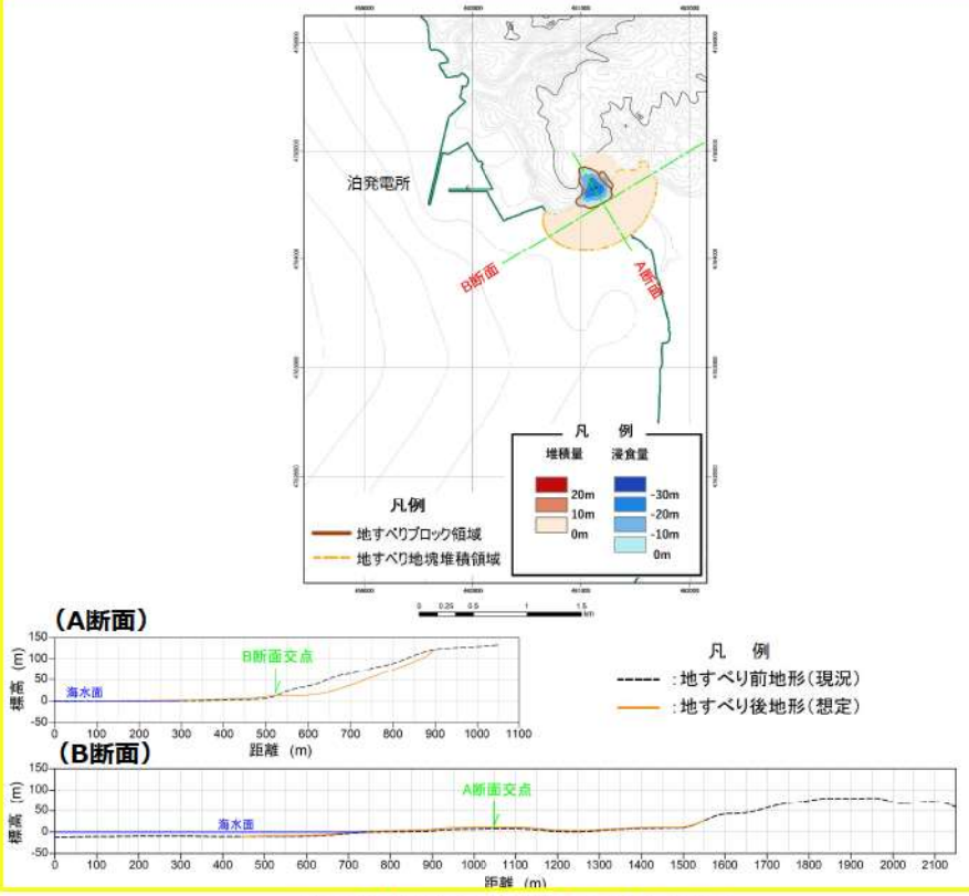
地滑り地形①による地形変化量
