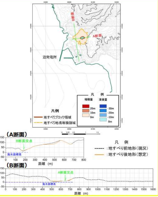
地滑り地形③による地形変化量
