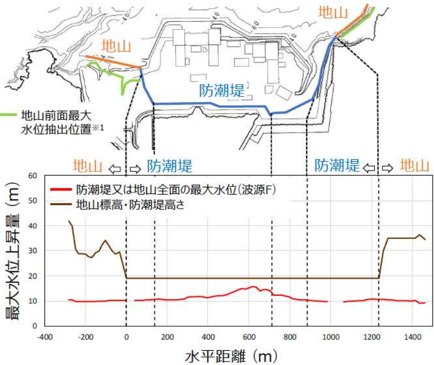
防潮堤沿いの最大水位縦断図 ※2※3 (基準津波は今後変更となる可能性あり)
