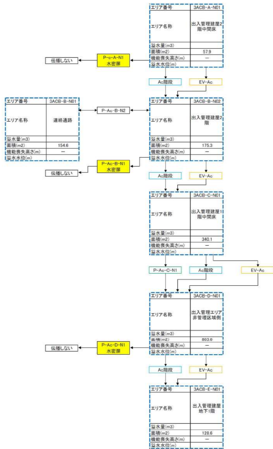
出入管理建屋 溢水伝播フロー図 (2/2)
