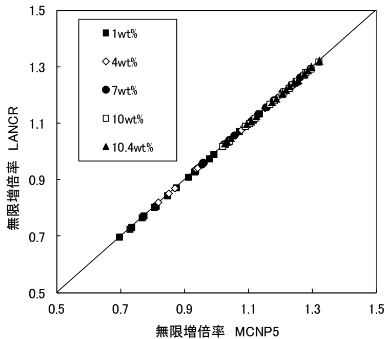
図 2-47 \text{PuF}_3 富化度ごとの無限増倍率の連続エネルギーモンテカルロ計算との比較
