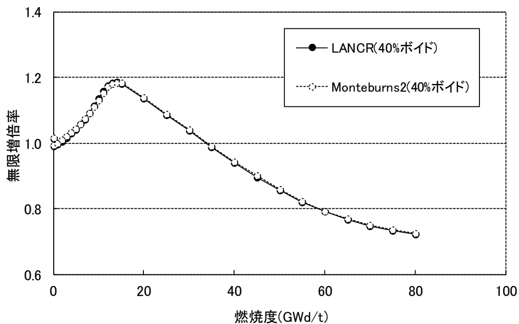
図 2-57 燃焼特性の連続エネルギーモンテカルロ計算との比較 (10×10 ウラン燃料集合体)
