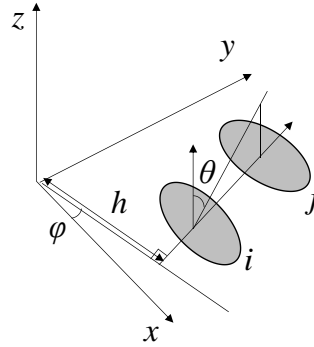
図 3.1-5 任意の2次元体系
