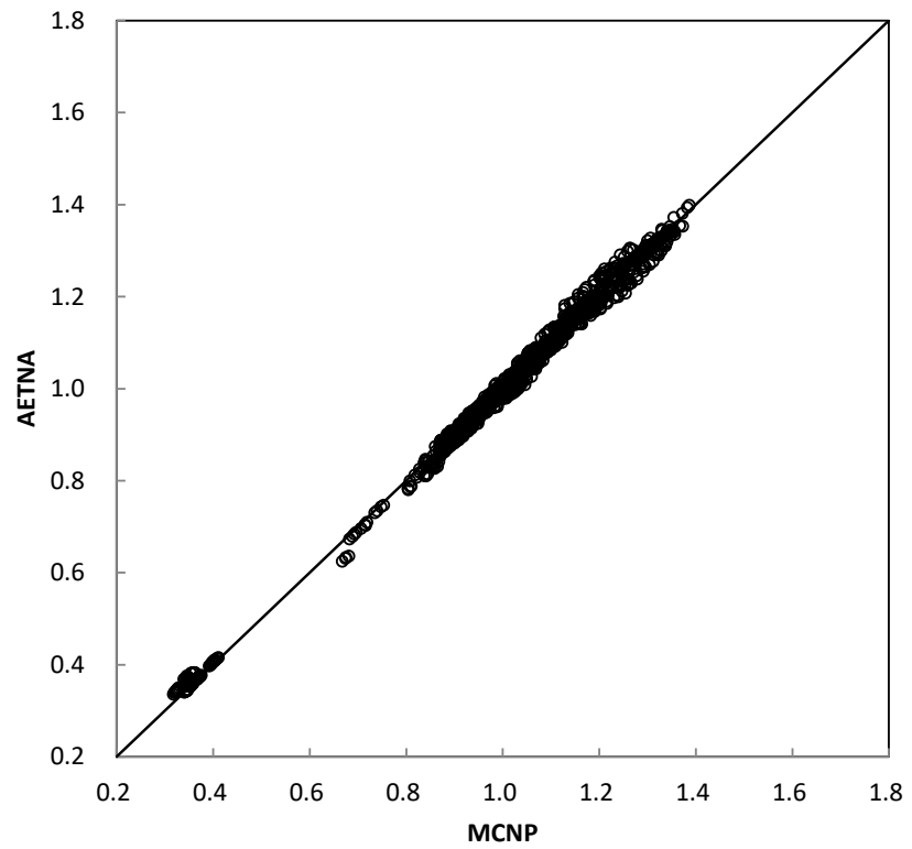
図 3-16 MOX 燃料混在炉心問題の全燃料棒の LPF の比較 (炉心 2)
