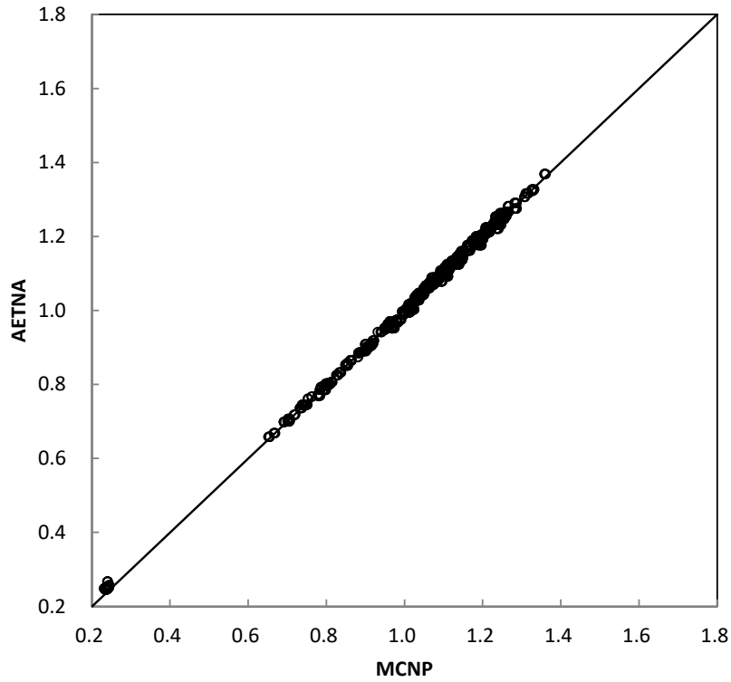
図 3-10 初装荷多種類燃料炉心問題の全燃料棒の局所出力分布の比較 (炉心 1)
