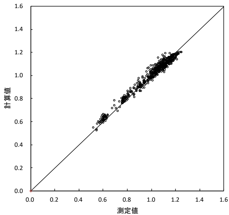
図 4.3-32 燃料棒ノーダル La-140 の計算値と測定値の比較 (集合体 2)
