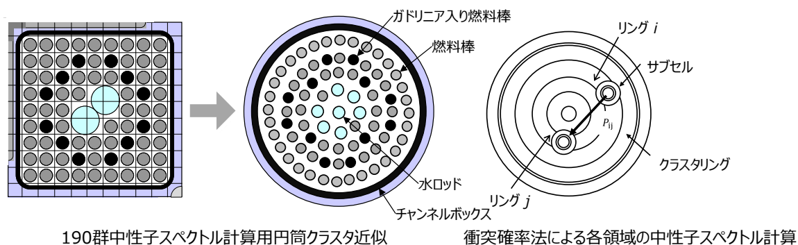
図 1. 4-3 円筒クラスタ近似による詳細エネルギー中性子スペクトル計算の概要
