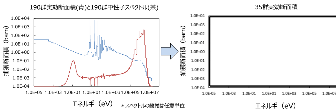
図 1. 4-4 中間エネルギー群（35 群）実効断面積の計算の概要
