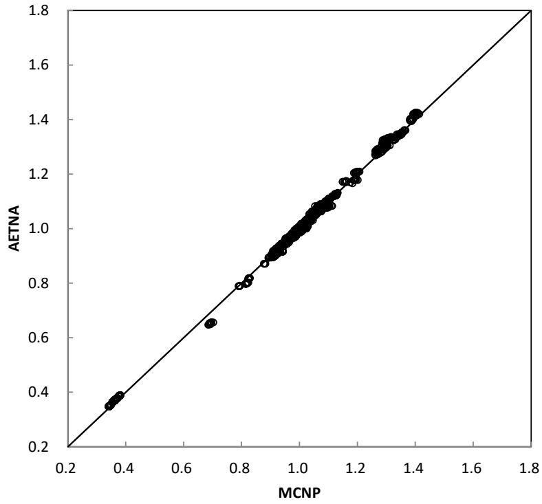
図 3-20 10×10 燃料平衡炉心問題の全燃料棒の局所出力分布の比較 (炉心 1)
