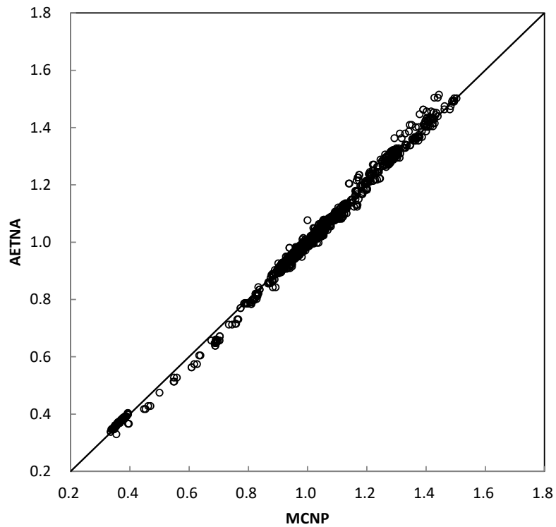
図 3-21 10×10 燃料平衡炉心問題の全燃料棒の局所出力分布の比較 (炉心 2)
