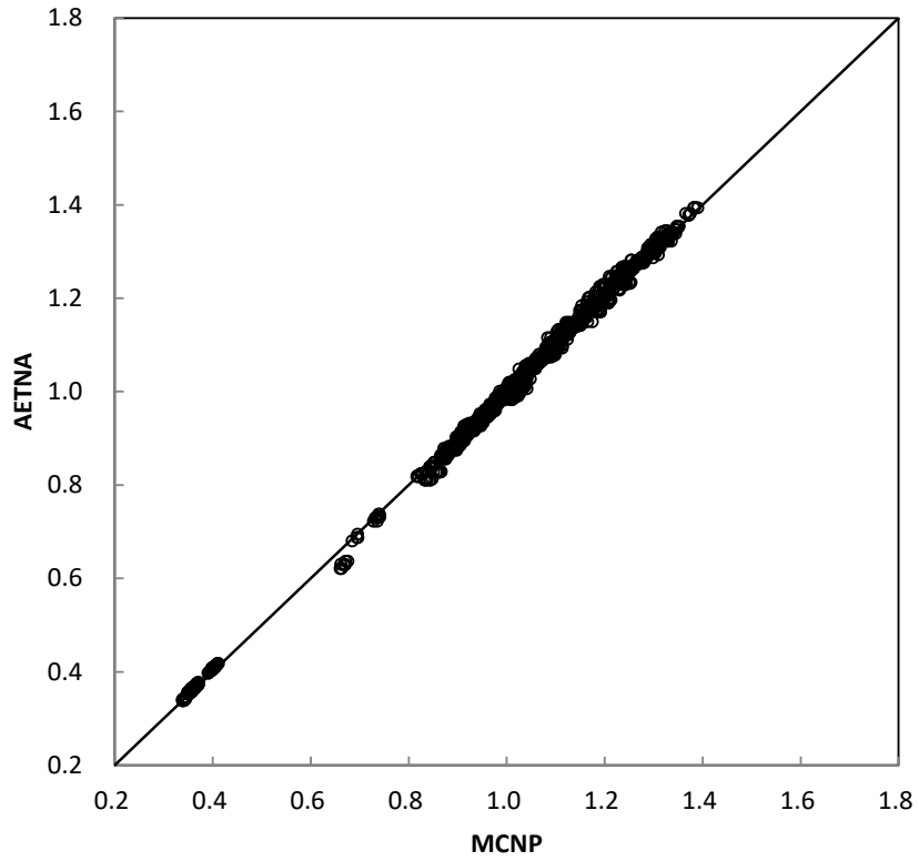
図 3-15 MOX 燃料混在炉心問題の全燃料棒の LPF の比較 (炉心 1)
