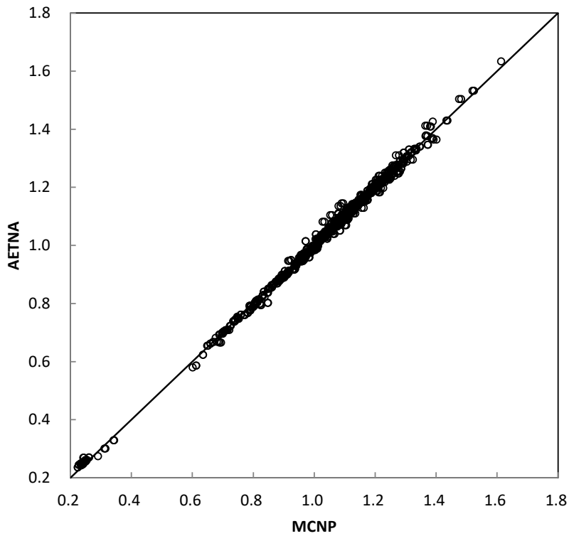
図 3-11 初装荷多種類燃料炉心問題の全燃料棒の局所出力分布の比較 (炉心 2)
