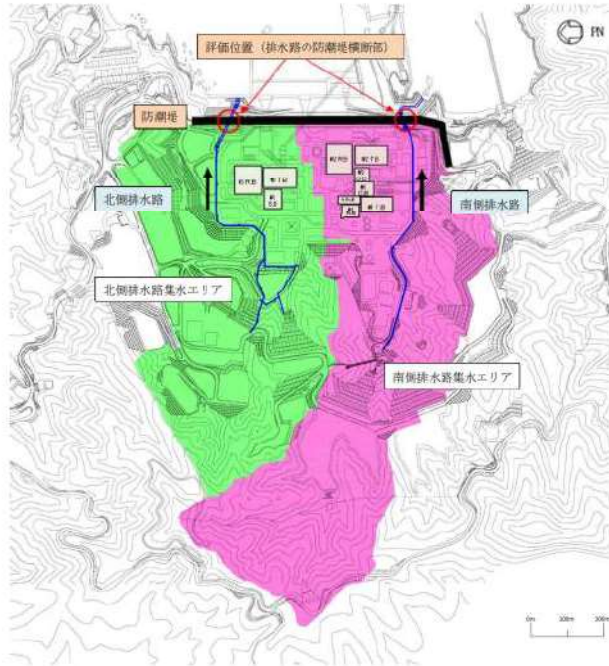
第1図 排水路の配置概要図
