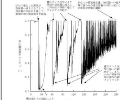
第5.2.2.7図 加圧器頂部クオリティの推移
