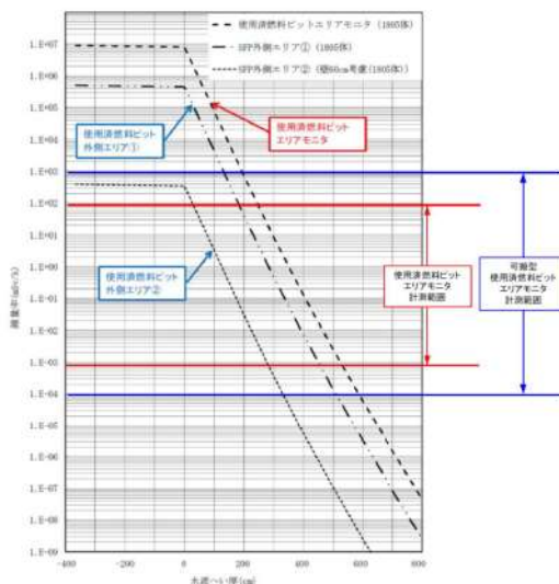
第9図 使用済燃料ピットの水遮蔽厚と線量率の相関図
