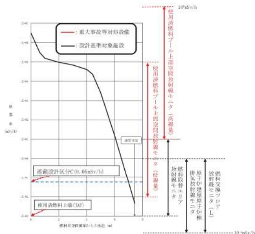
図54-11-8 水位と放射線量率の関係
