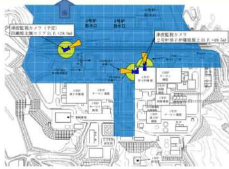
図2.1-4 2号炉原子炉施設と津波監視カメラの監視可能な範囲
