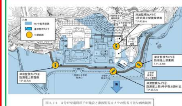
図2.1-4. 3号炉発電用原子炉施設と津波監視カメラの監視可能な範囲
