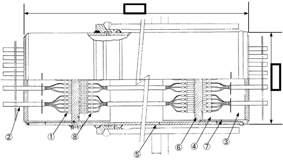
ピッグテイル型電気ペネトレーション構造図 [ ] 製
