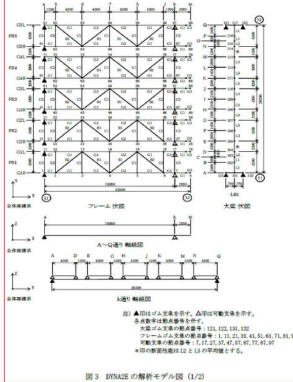
図3 DYNAGEの解析モデル図 (1/2)
