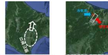
第2.2.5.5.2図 親雲の発生箇所と移動方向 (左) 及び竜巻の発生箇所 (右) ※ ※: 軽水型原子力発電所の竜巻影響評価における設計竜巻風速及び飛来物速度の設定に関するガイドライン, 日本保全学会, 原子力規制関連事項検討会, 2015
