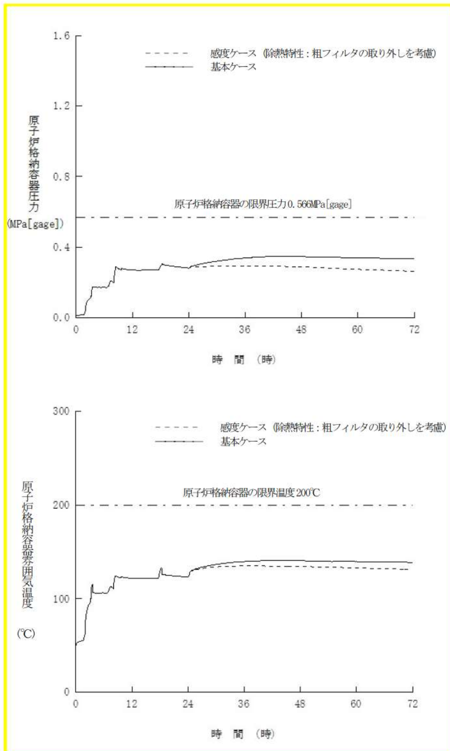
図4 雰囲気圧力・温度による静的負荷 (格納容器過温破損)
