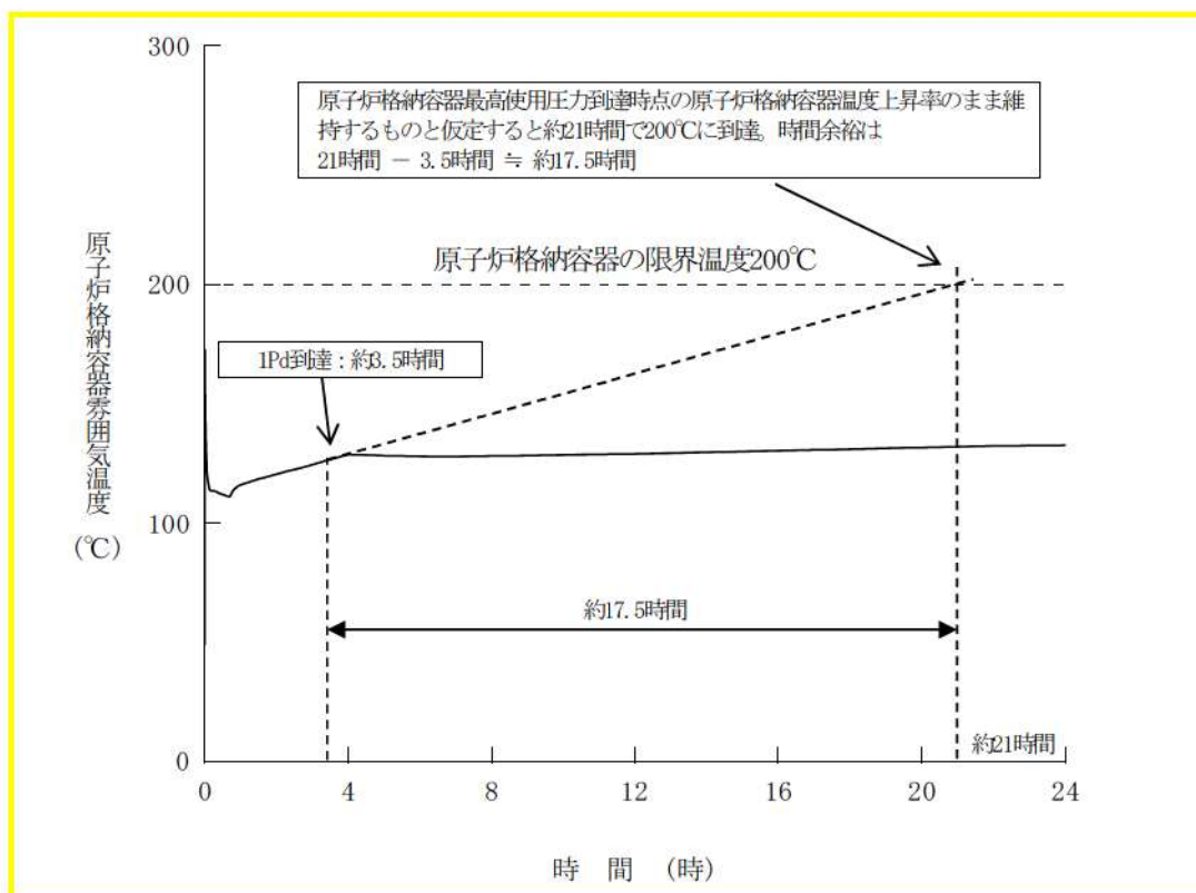
図2 原子炉格納容器雰囲気温度の推移
