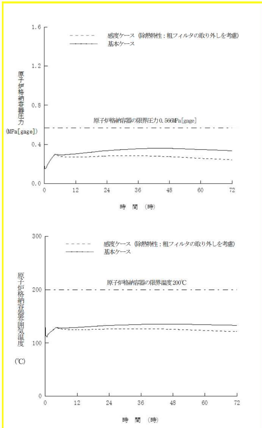
図2 原子炉格納容器の除熱機能喪失
