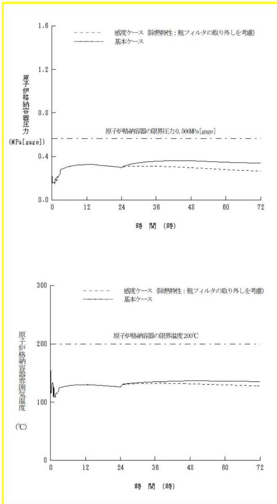
図3 雰囲気圧力・温度による静的負荷 (格納容器過圧破損)
