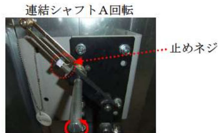
ダンパ駆動部写真
