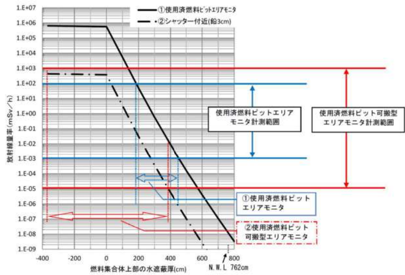
第 27 図 使用済燃料ピットの遮蔽厚と放射線量率の相関図
