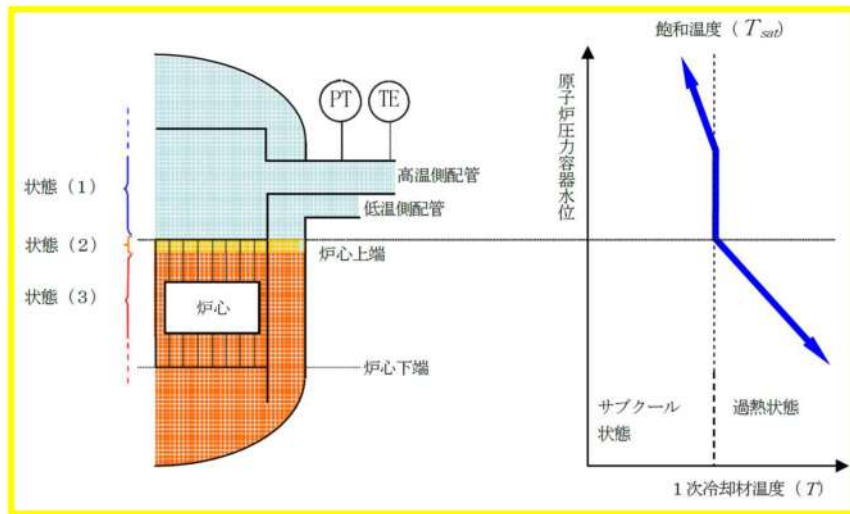
第5図 原子炉圧力容器内の水位と水位変化の概念図
