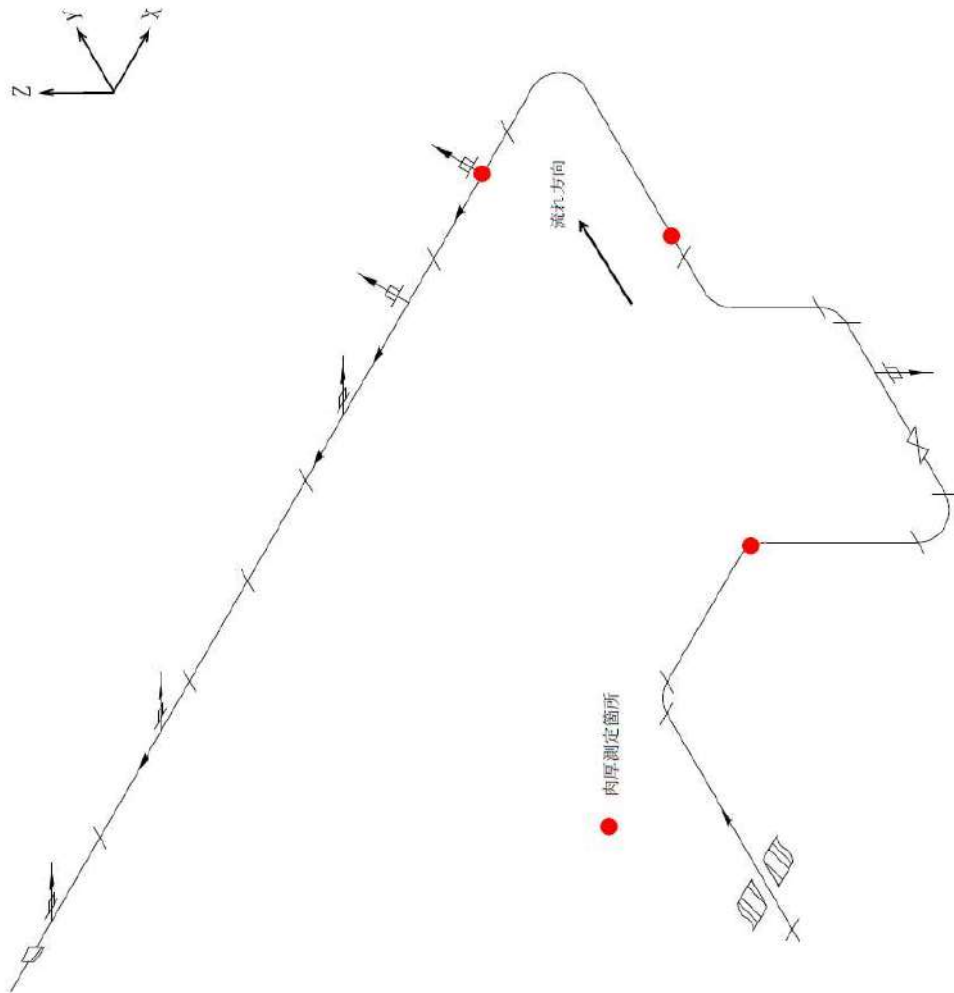
図1 肉厚測定箇所（水消火系）（1/5）
