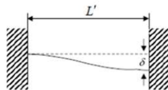
両端固定の例
